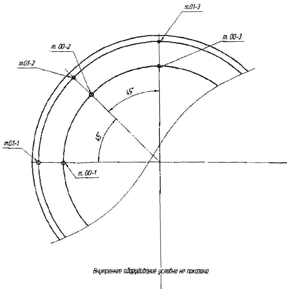
Рисунок А.4 – Схема измерений нижней части резервуара
