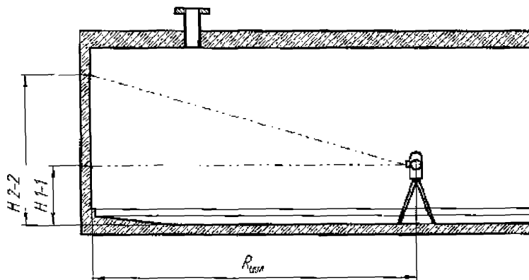
Рисунок А.3 – Схема измерений диаметра резервуара
