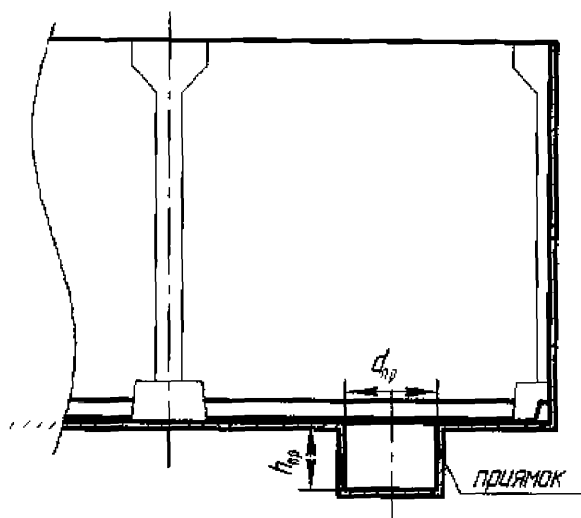
Рисунок А.5 Схема измерений параметров призмка
