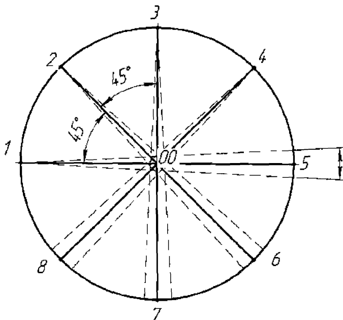
Рисунок А.2 – Схема определения центра дна резервуара
