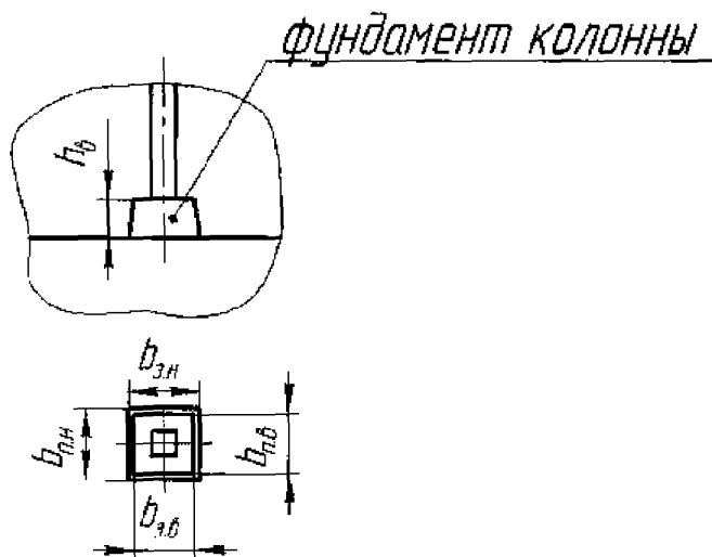
Рисунок А.6 – Схема измерений параметров фундамента колонны
