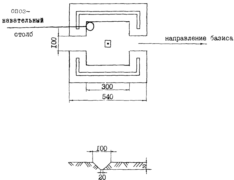
Рис. 2. Внешнее оформление базисных центров 2-го разряда (размеры даны в см)
