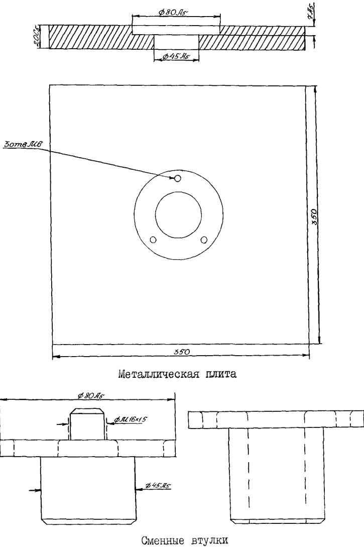
Рис. 4. Устройство для принудительного центрирования (размеры даны в мм)
