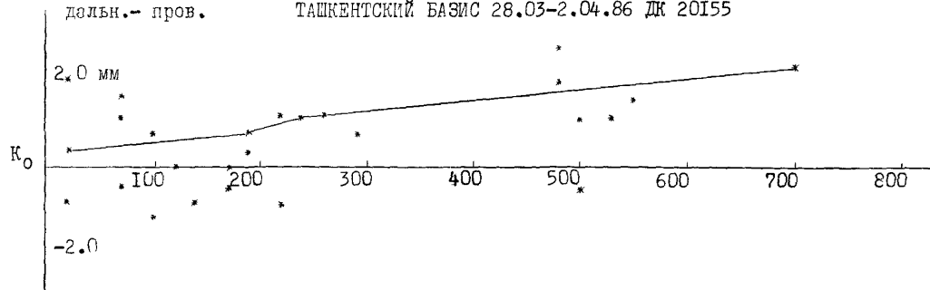
дальн.- пров. ГРАФИК ПРИБОРНОЙ ПОПРАВКИ "К" ("УРАВНЕНИЕ ДАЛЬНОМЕРА") ТАШКЕНТСКИЙ БАЗИС 28.03-2.04.86 ДК 20155
