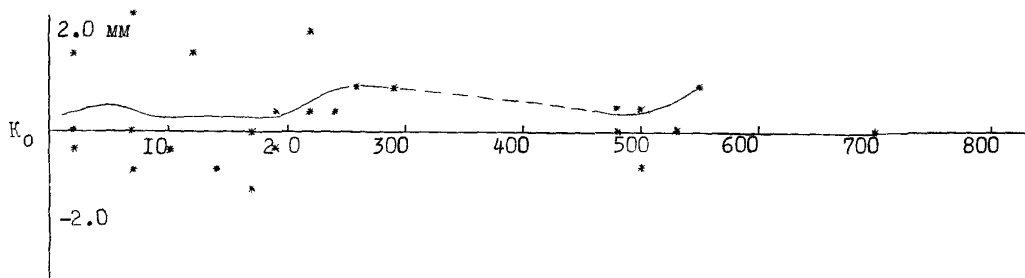
дальн.- пров. ГРАФИК ПРИБОРНОЙ ПОПРАВКИ "К" ("УРАВНЕНИЕ ДАЛЬНОМЕРА") ТАШКЕНТСКИЙ БАЗИС 28.03-2.04.86 ДК 20155
