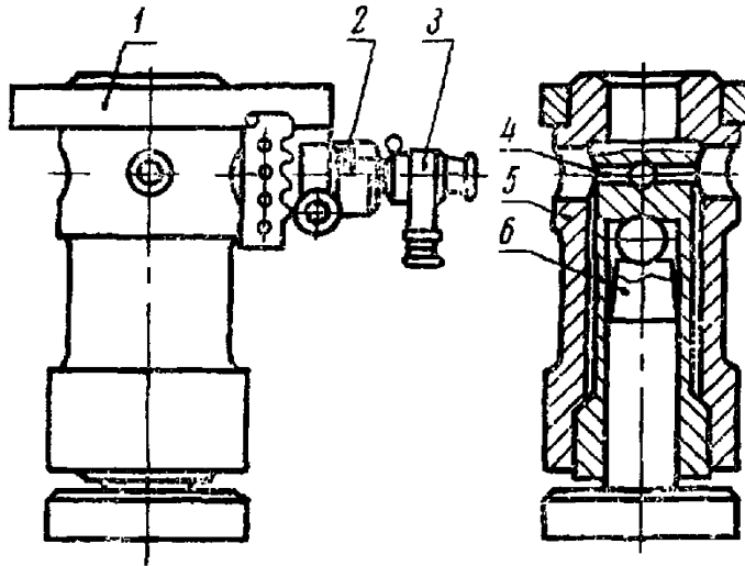
Черт. 1. Схема устройства динамометра ДОЖ
