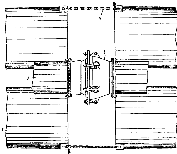
Рис. 7. Шарнирное соединение звеньев
