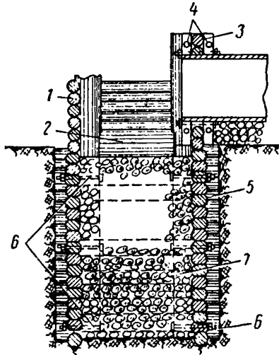
Рис. 12. Колодец на ряжевом основании
