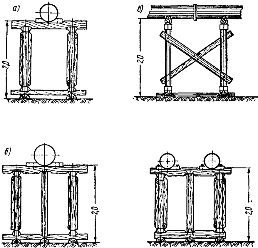
Рис. 18. Рамные опоры
