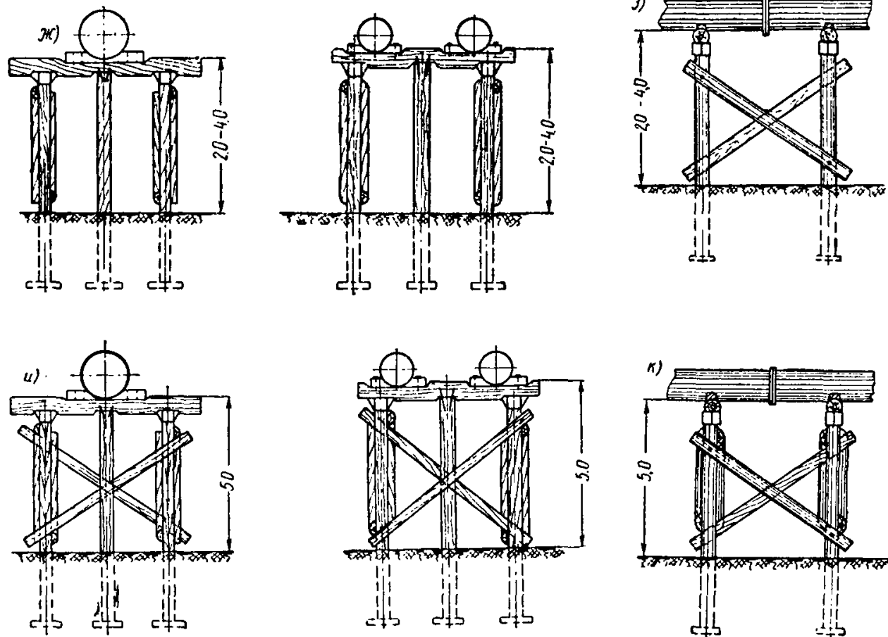
Рис. 16. Закопные опоры
