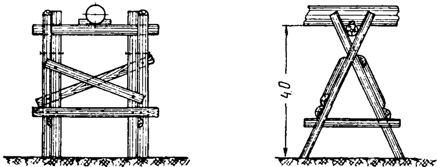
Рис. 19. Козловая опора
