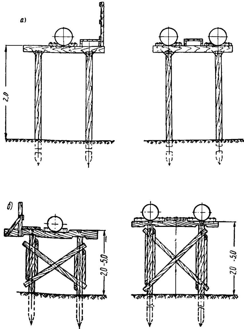
Рис. 17. Свай
