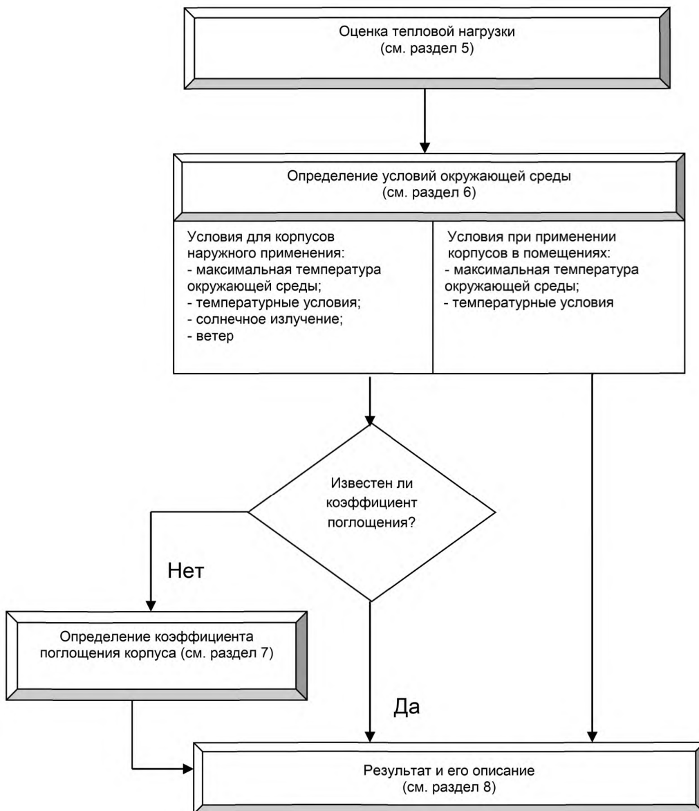
Рисунок 2 — Технологическая схема для определения коэффициента поглощения
