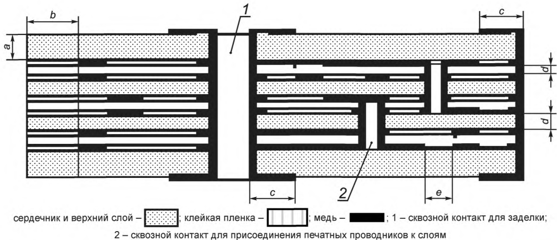
Рисунок 2 – Минимальные расстояния для многослойных печатных монтажных плат.
