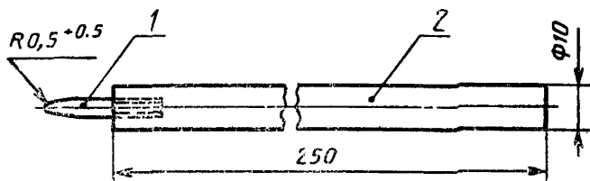
1 — пластмассовый наконечник; 2 — сталь Черт. 3
