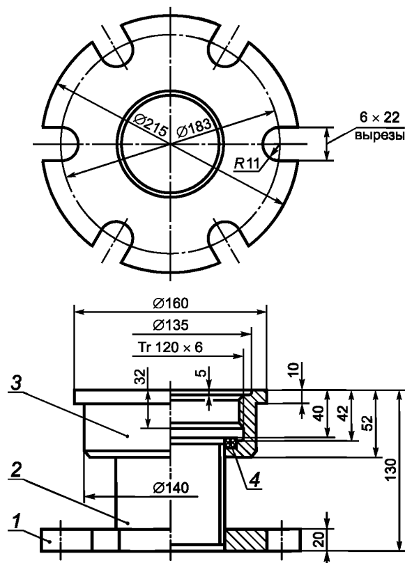
Рисунок 11 — Переходной патрубок DN 80 типа 4 для нефтеводной смеси
