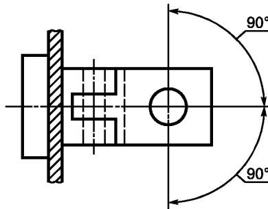
Рисунок 5 — Минимальные углы поворота сцепного устройства
