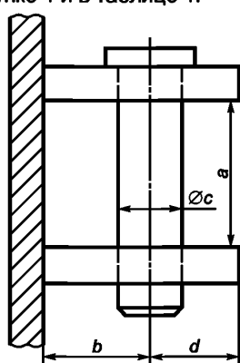
а — сцепное устройство с шкворнем
