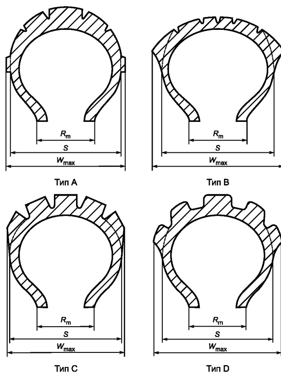
Рисунок 1 — Типы протектора шин
