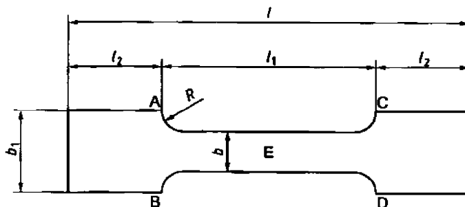
Рисунок 1— Форма испытуемого образца
