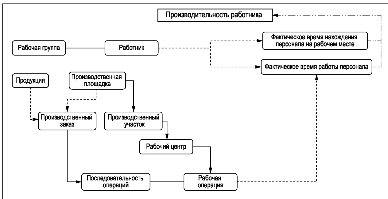
Рисунок А.1 — Диаграмма модели действия элементов KPI-показателя «Производительность работника»
