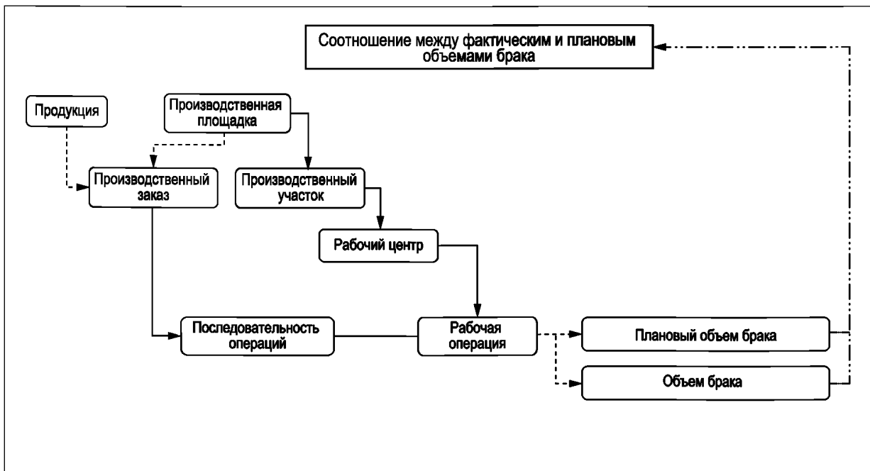
Рисунок А.14 — Диаграмма модели действия элементов КРІ-показателя «Соотношение между фактическим и плановым объемами брака»
