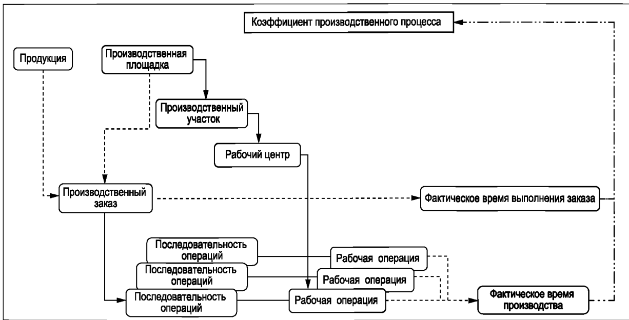
Рисунок А.13 — Диаграмма модели действия элементов КРІ-показателя «Кoeffициент производственного процесса»
