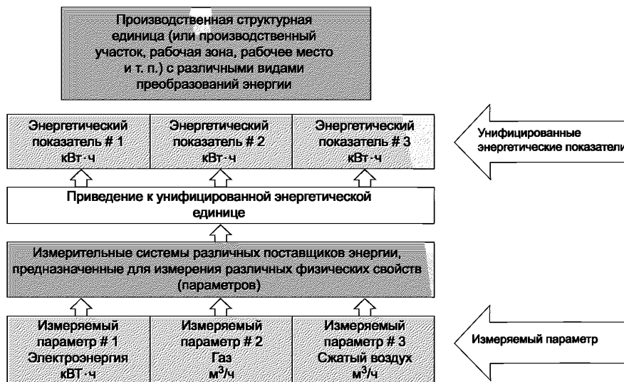
Рисунок 7 — Преобразование измеренных параметров в энергетические единицы
