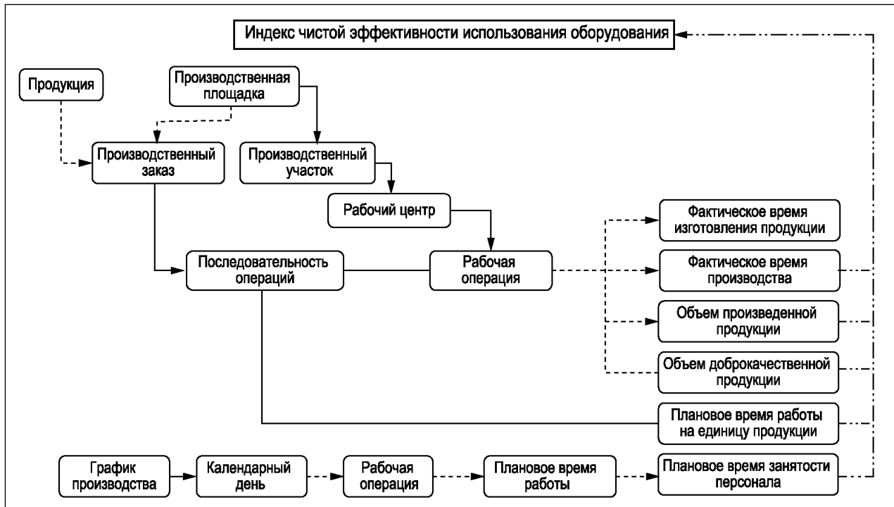
Рисунок А.7 — Диаграмма модели действия элементов KPI-показателя «Индекс чистой эффективности использования оборудования (NEE)»
