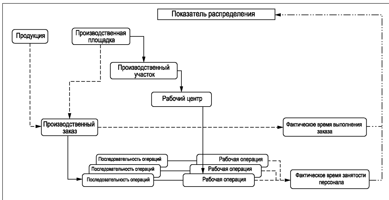
Рисунок А.2 — Диаграмма модели действия элементов KPI-показателя «Показатель распределения»
