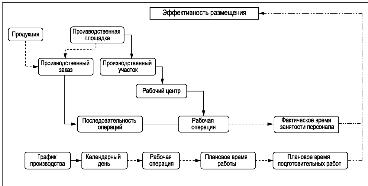
Рисунок А.4 — Диаграмма модели действия элементов КPI-показателя «Эффективность размещения»
