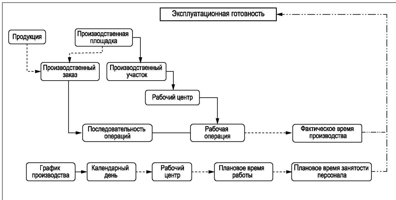
Рисунок А.8 — Диаграмма модели действия элементов KPI-показателя «Эксплуатационная готовность»
