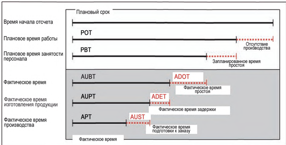
Рисунок 4 — Временные диаграммы рабочих операций
