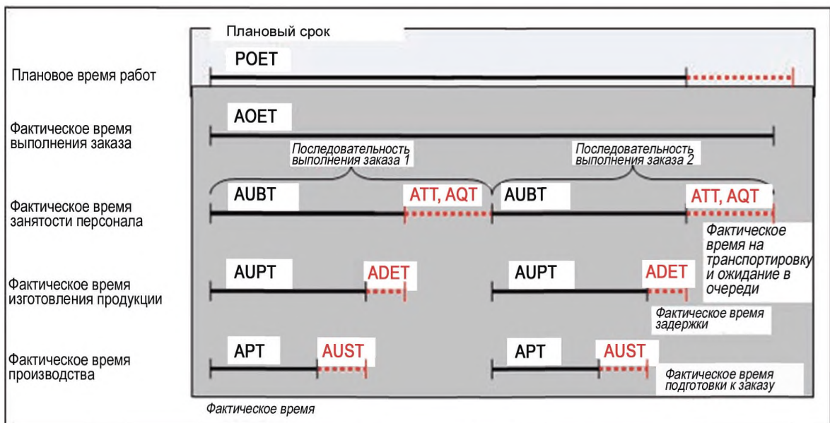
Рисунок 5 — Временные диаграммы работ по производственному заказу
