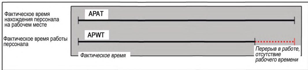
Рисунок 6 — Временные диаграммы персонала
