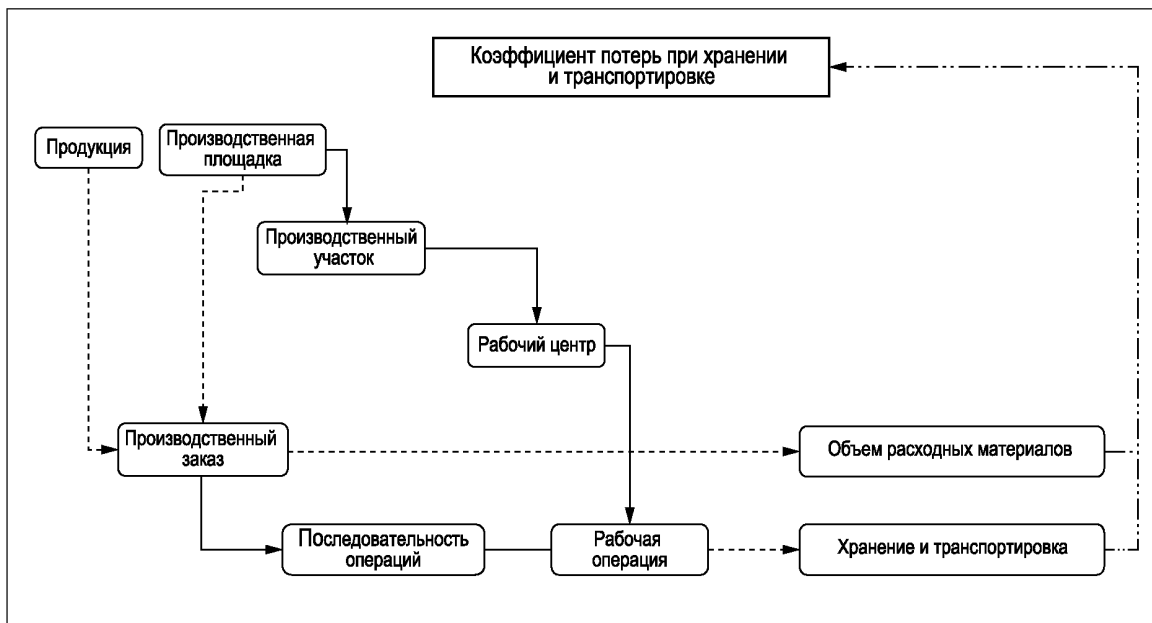
Рисунок А.26 — Диаграмма модели действия элементов КPI-показателя «Коэффициент потерь при хранении и транспортировке»
