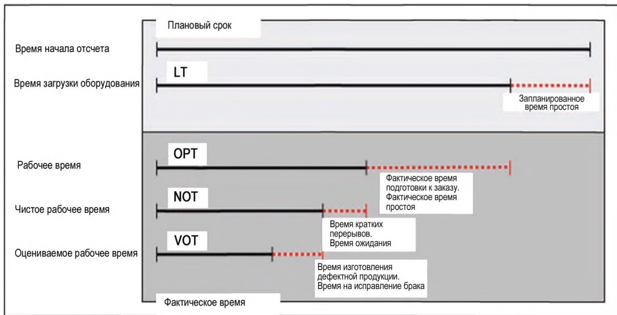
Рисунок В.1 — Временная модель для расчета общей эффективности использования оборудования (ОЕЕ)
