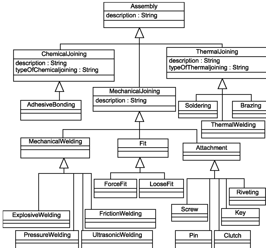
Рисунок В.13 — Объектная модель AssemblyProcess
