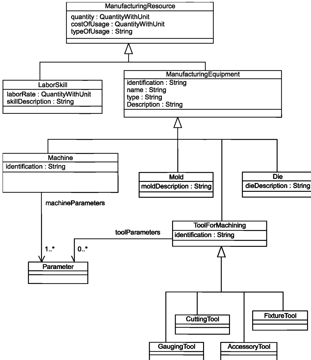
Рисунок В.14 — Объектная модель ManufacturingResource
