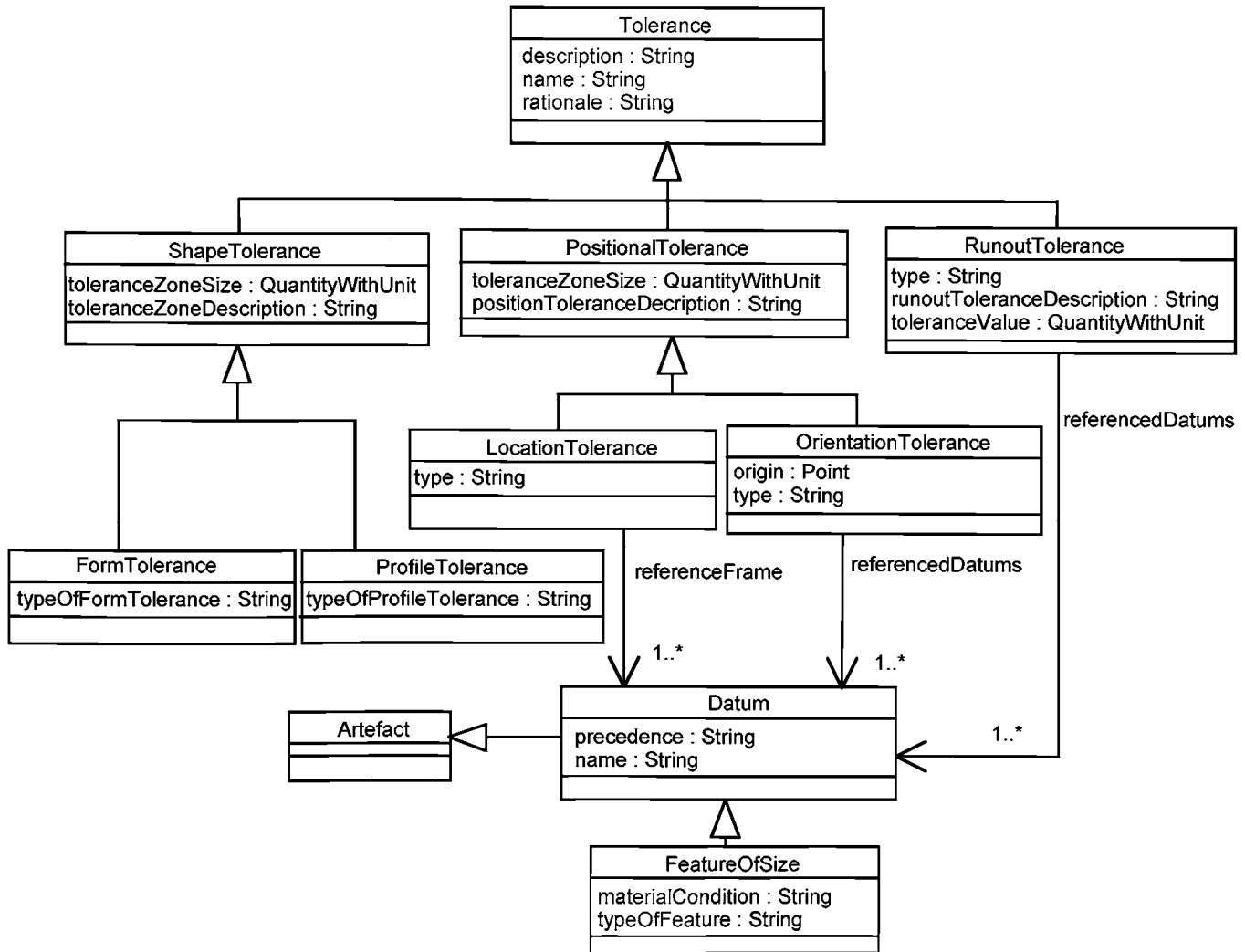
Рисунок В.4 — Диаграмма класса Tolerance
