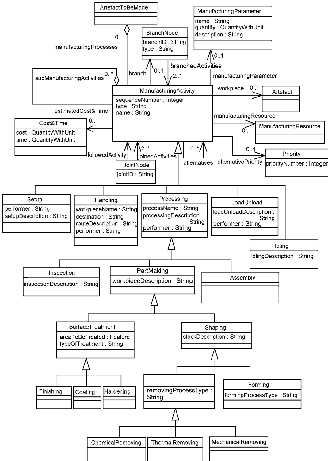
Рисунок В.10 — Диаграмма класса ManufacturingProcess
