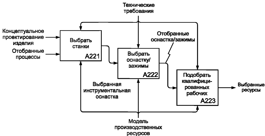
Рисунок В.9 — Выбор производственных ресурсов
