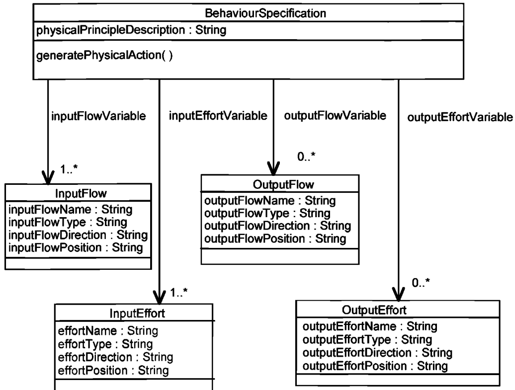
Рисунок В.6 — Диаграмма класса Behaviour
