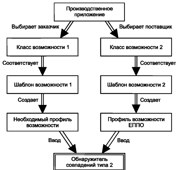
Рисунок 4 — Классы возможностей одного производственного приложения
