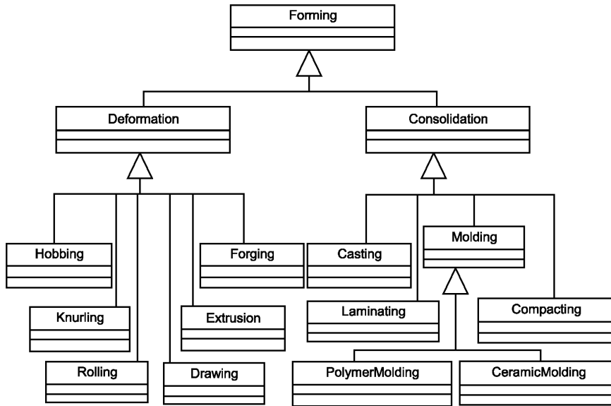
Рисунок В.12 — Модель процесса придания формы
