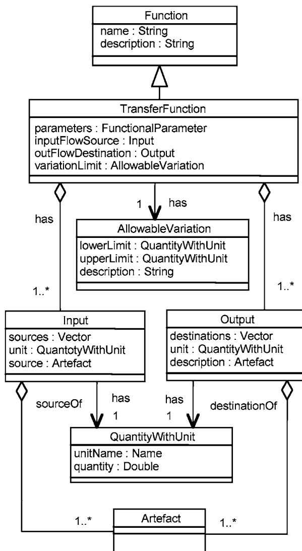
Рисунок В.5 — Диаграмма класса Function
