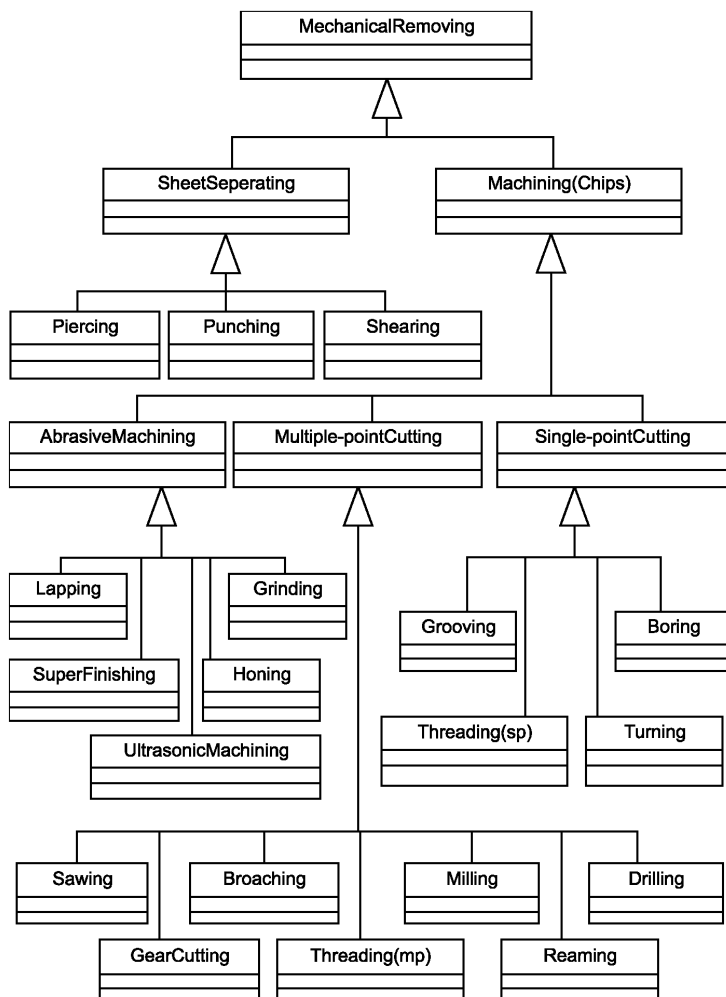
Рисунок В.11 — Объектная модель процесса MechanicalRemoving
