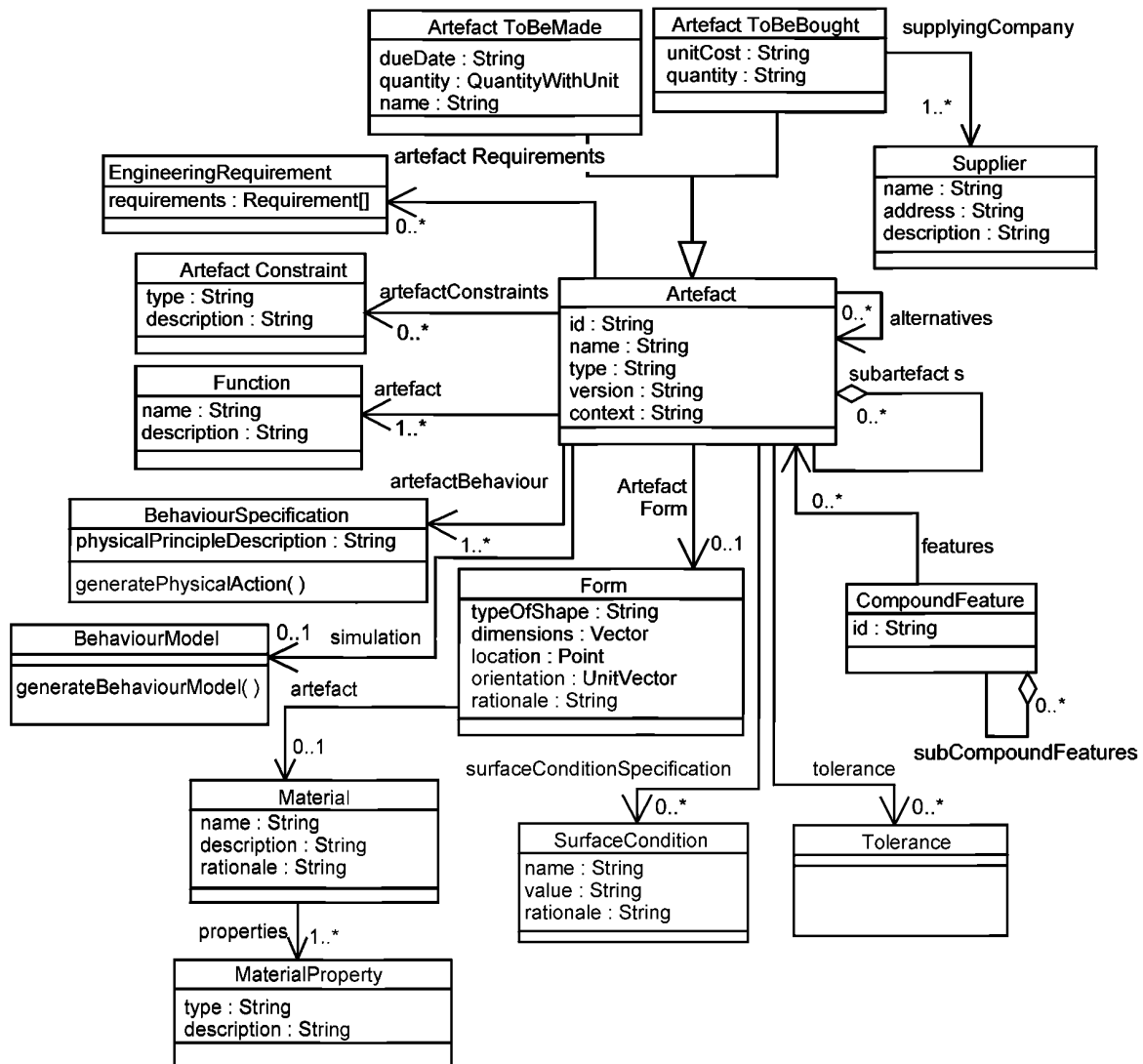
Рисунок В.3 — Диаграмма класса Artefact
