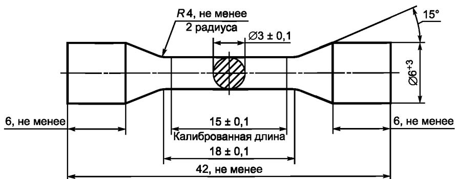
Рисунок 1 — Образец с короткой головкой
