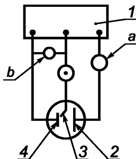
1 — потенциостат; 2 — противоэлектрод; 3 — контрольный электрод; 4 — рабочий электрод; a — измерение тока; b — измерение потенциала
