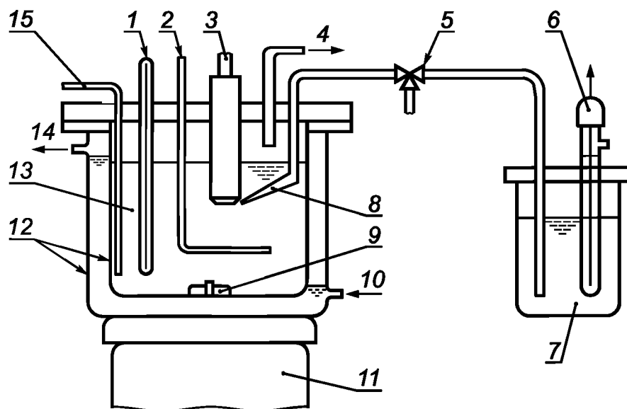
1 — термометр; 2 — противоэлектрод; 3 — рабочий электрод; 4 — выход газов; 5 — электролитический мостик; 6 — контрольный электрод (насыщенный хлоридом серебра, НХС); 7 — насыщенный раствор KCl; 8 — капилляр; 9 — магнитная мешалка, покрытая тефлоном; 10 — вход для воды; 11 — мотор для магнитной мешалки; 12 — сосуд с двойными стенками; 13 — раствор электролита; 14 — выход для воды; 15 — барботер (использующий азот)
