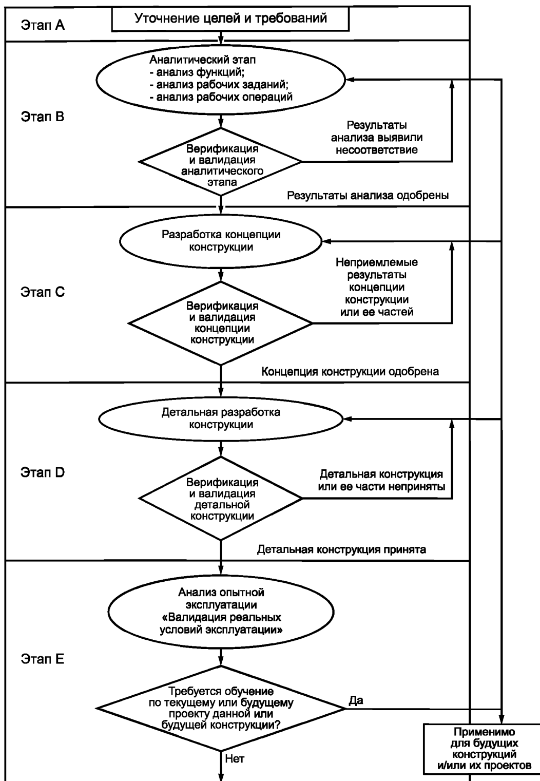
Рисунок 2 — Верификация и валидация при проектировании
