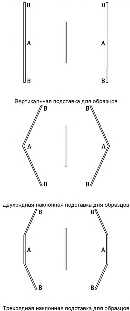
Рисунок В.1 — Определение равномерности энергетической освещенности в устройствах для экспонирования, использующих вращающуюся подставку для образцов
