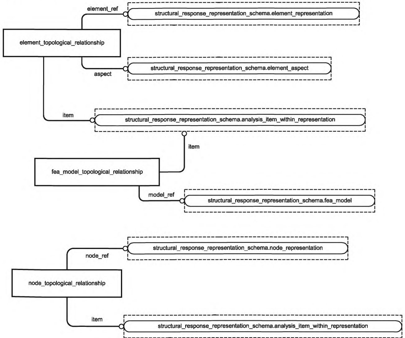
Рисунок D.11 — Представление схемы fea_definition_relationships_schema в формате EXPRESS-G (диаграмма 3 из 3)
