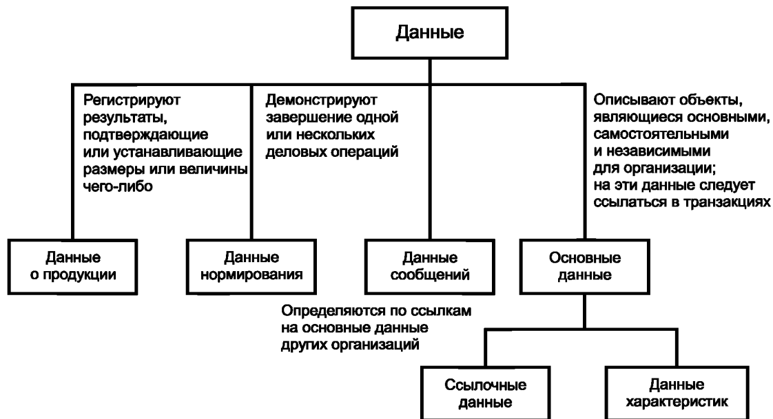
Рисунок 1 — Таксономия данных
