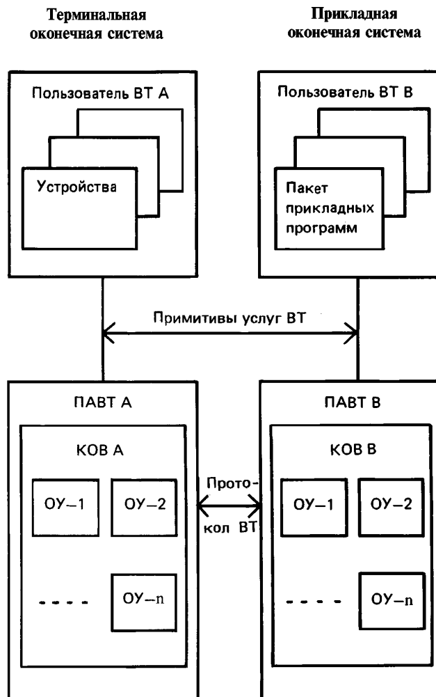
Рисунок 2 — Объекты управления в модели протокола ВТ
