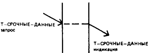
Рисунок 3 — Временные диаграммы примитивов услуг транспортного уровня (лист 1)
