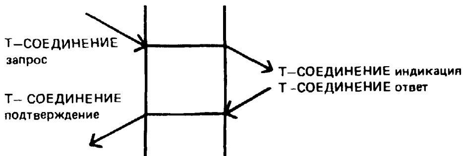
Рисунок 5 — Последовательность примитивов при успешном установлении СТУ
