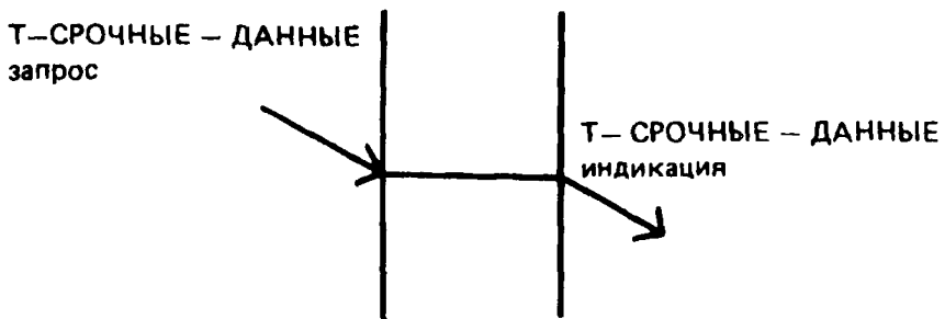
Рисунок 7 — Последовательность примитивов при успешной передаче срочных данных
