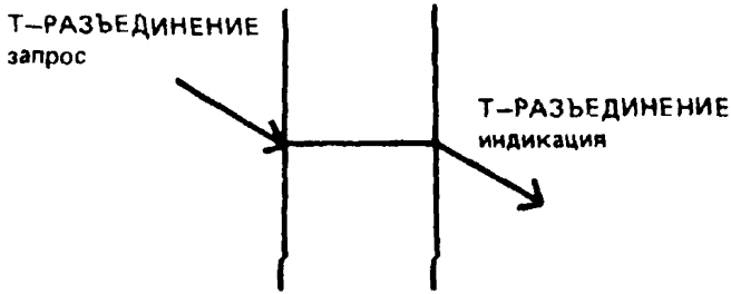
Рисунок 8 — Последовательность примитивов при разъединении СТУ по инициативе пользователя УТУ
