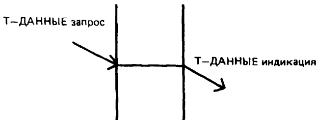
Рисунок 6 — Последовательность примитивов при успешной передаче данных
