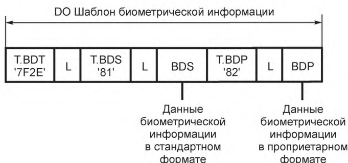
Рисунок С.1 — Шаблон биометрических данных в поле данных команды (примеры)
