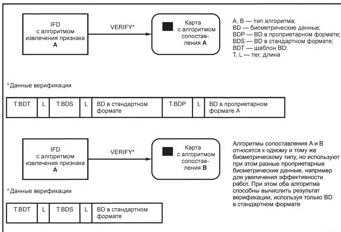
Рисунок 1 — Использование биометрических данных со стандартной и проприетарной структурами
