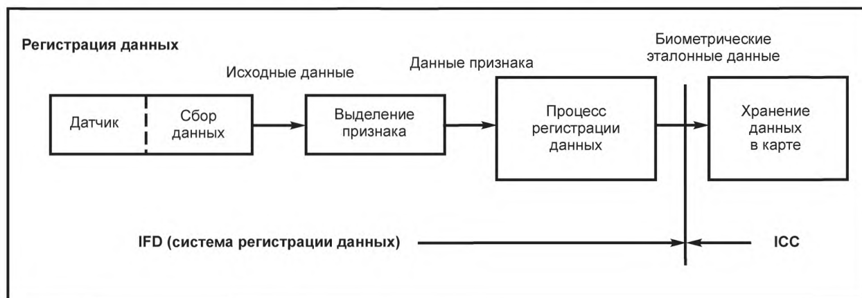
Рисунок А.1 — Общая схема процесса регистрации данных
