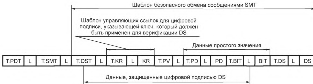
Рисунок D.4 — Шаблон персональных данных с BIT, защищенных цифровой подписью (пример)
