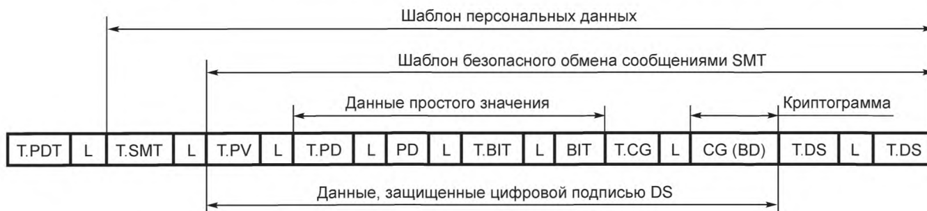
Рисунок D.5 — Шаблон персональных данных, защищенный цифровой подписью и содержащий помимо DO криптограмму для биометрических данных (пример)
