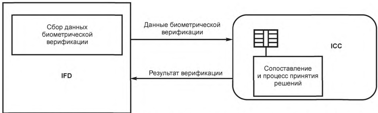
Рисунок А.5 — Сценарий с сопоставлением и процессом принятия решений внутри карты
