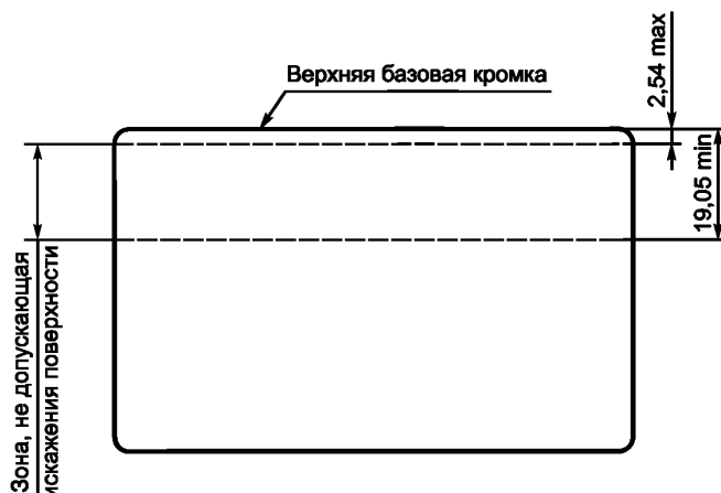
Рисунок — Зона на карте с магнитной полосой, где не допускаются искажения поверхности
