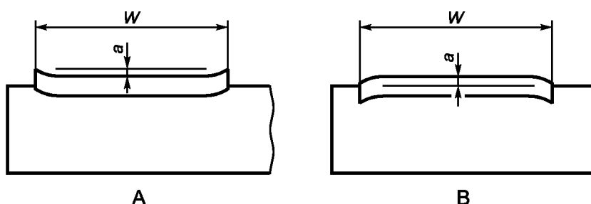
Рисунок 3 — Профиль поверхности
