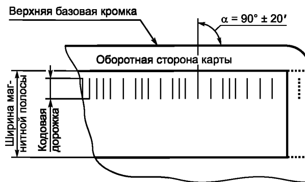
Рисунок 8 — Угол записи
