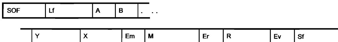
Рисунок E.9 — Синтаксическая структура заголовка кадра
