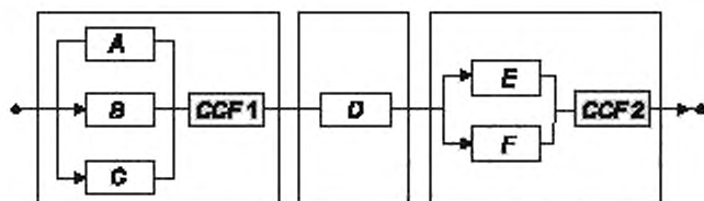
Рисунок Б.1 — Блок-схема надежности полного контура безопасности
