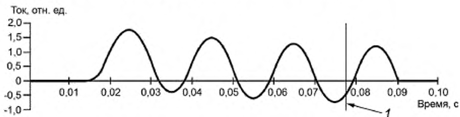
в) Третья операция (при среднем времени дуги)
