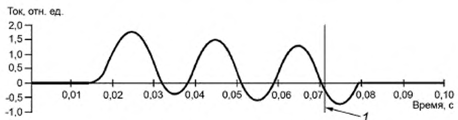
а) Первая операция (при минимальном времени дуги)
