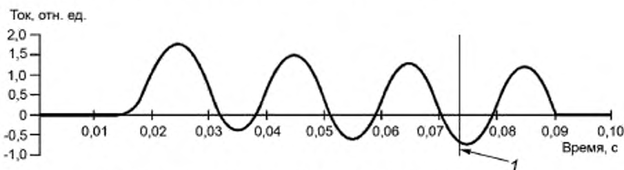
б) Вторая операция (при максимальном времени дуги)
