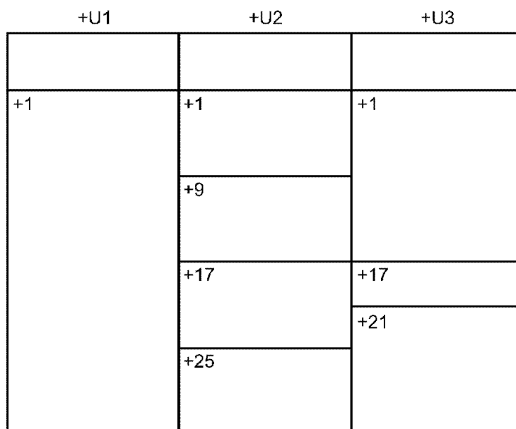
Рисунок Н.5 — Компоновочный чертеж местоположений ЩСУ =G1=W1
