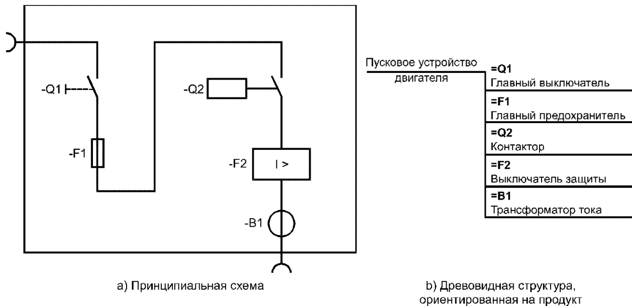
Рисунок Н.6 — Пусковое устройство двигателя
