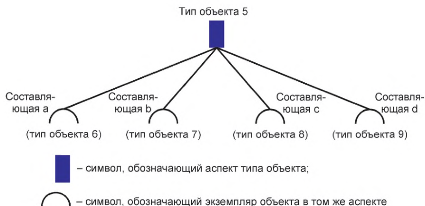
Рисунок 12 — Составляющие типа объекта 5 в одном аспекте
