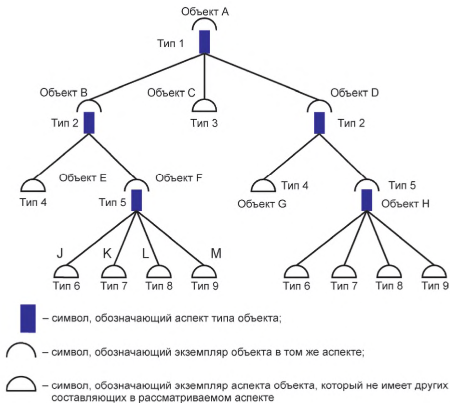
Рисунок 13 — Древовидная структура типа объекта 1
