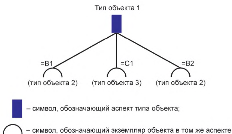
Рисунок G.1 — Функционально-ориентированная структура типа объекта 1
