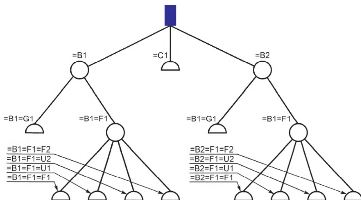
Рисунок G.3 — Функционально-ориентированная структура типа объекта 5
