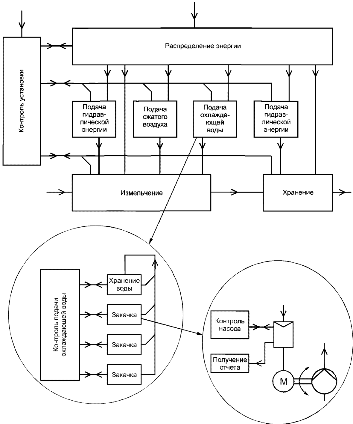
Рисунок 14 — Функционально-ориентированная структура
