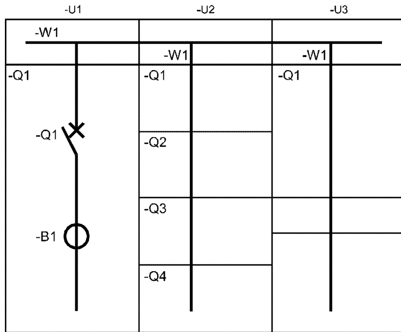
Рисунок Н.4 — Компоновочный чертеж компонентов ЩСУ =G1=W1
