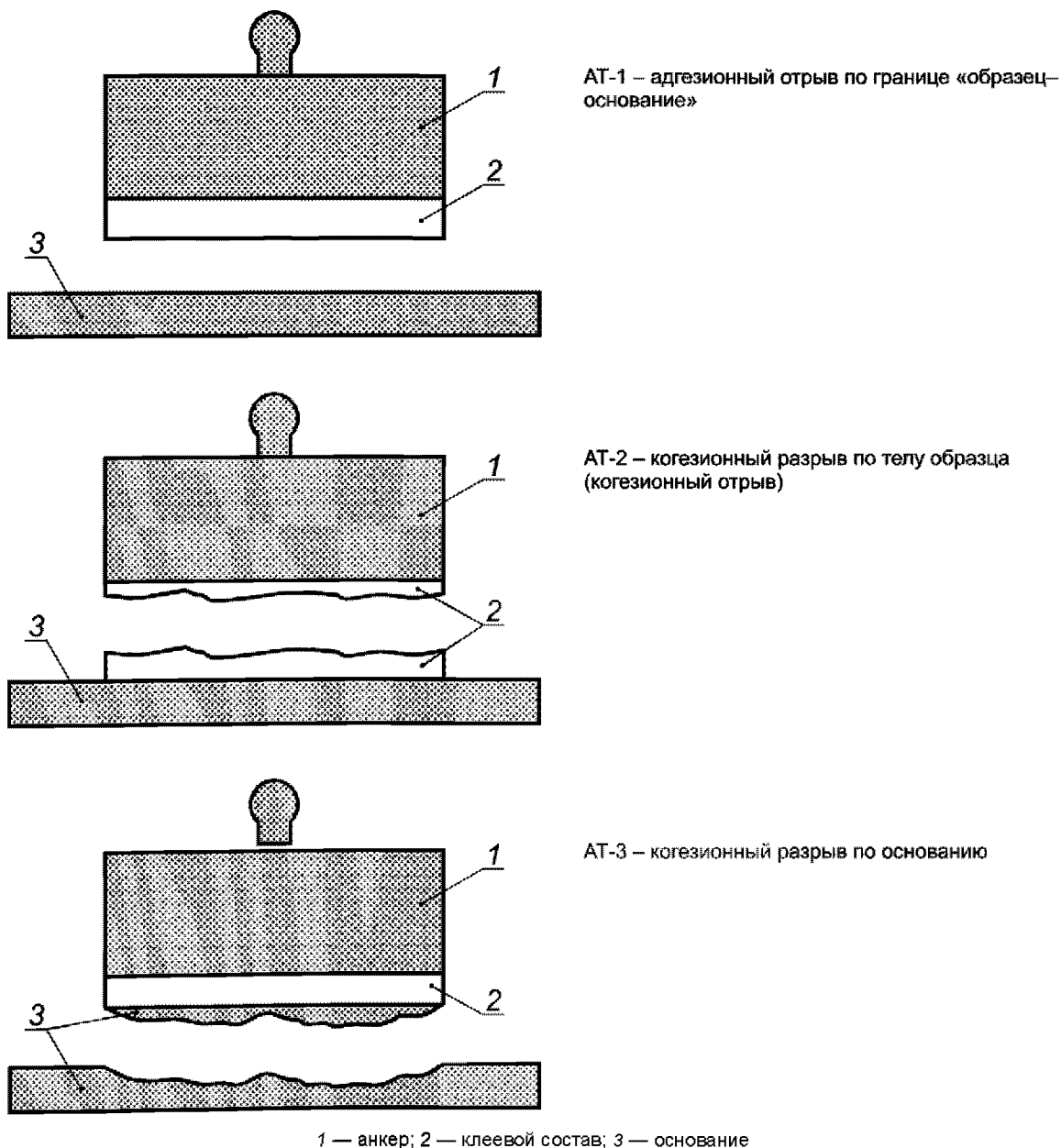
Рисунок 1 — Основные характерные виды отрыва образцов при определении прочности сцепления с основанием
