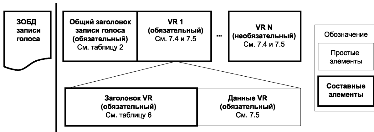
Рисунок 4 — Структура XML-элементов
