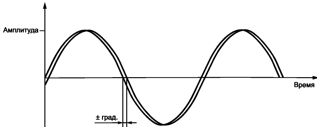
Рисунок В.1 — Фазовая модуляция колебаний (PJM)
