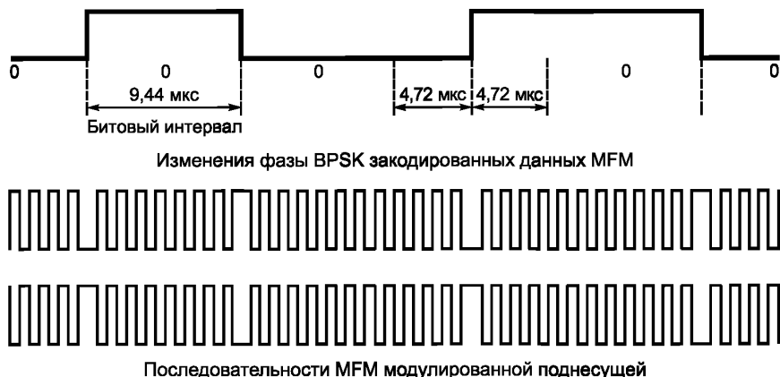
Рисунок 38 — Метод PJM: MFM кодирование ответа и временная диаграмма двоичной последовательности 000100
