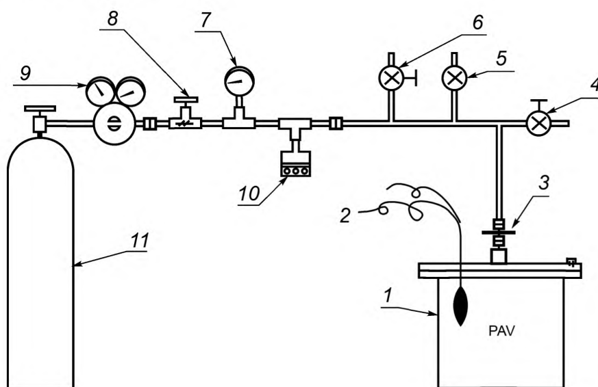
1 — камера высокого давления; 2 — температурный датчик; 3 — быстросъемное соединение; 4, 8 — игольчатый клапан; 5 — разгрузочный клапан; 6 — воздуховыпускной клапан; 7 — манометр; 9 — регулятор давления; 10 — предохранительная разрывная диафрагма; 11 — сжатый воздух
