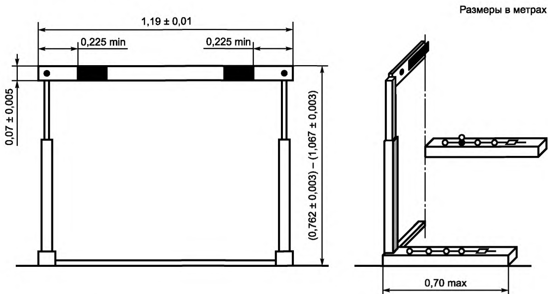
Рисунок 1 — Основные размеры элементов конструкции барьера для бега
