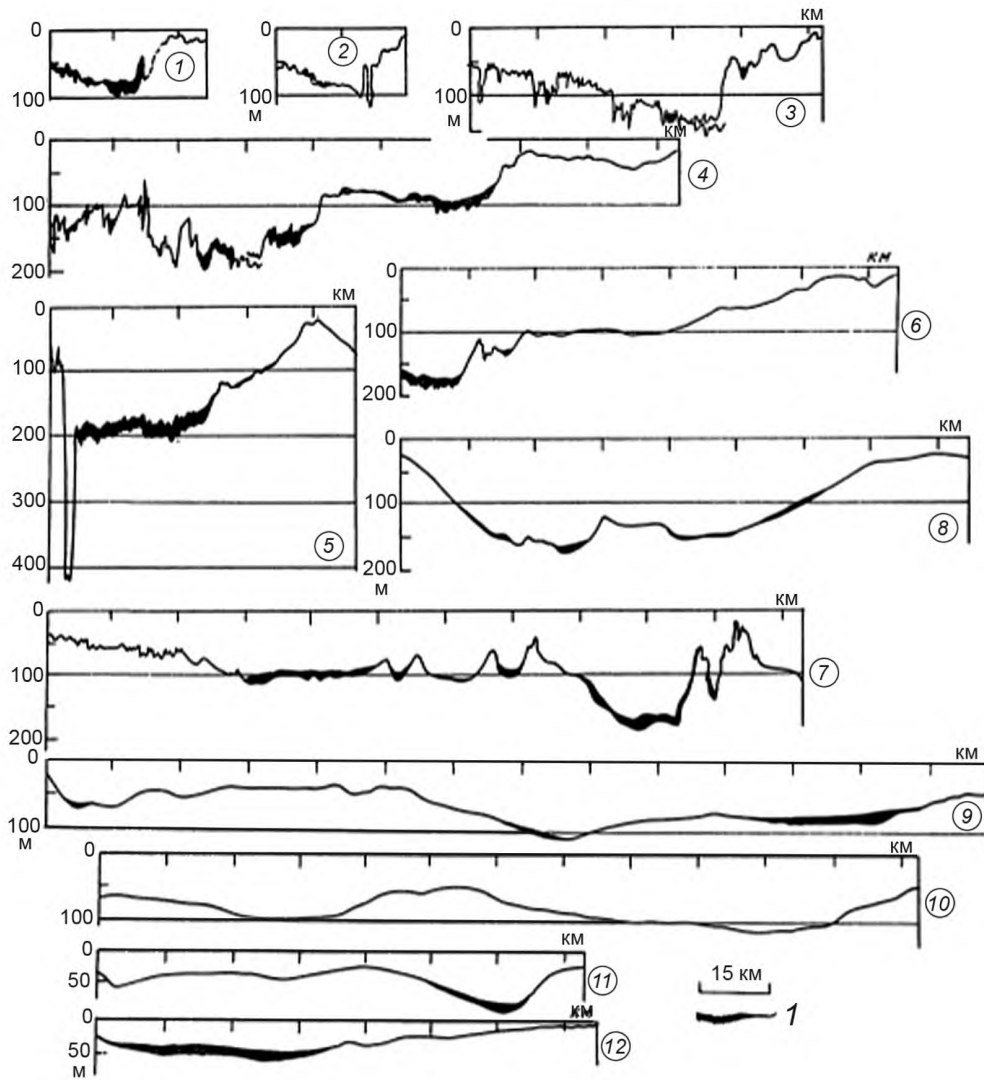
б) Профили рельефа дна Балтийского моря
