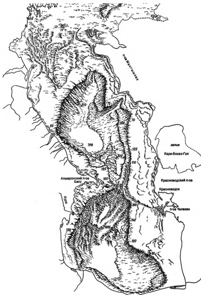
Рисунок В.2 — Физиографическая карта Каспийского моря
