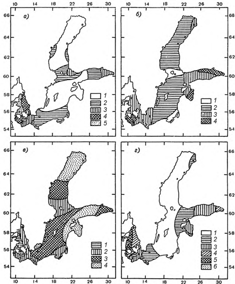
а — суммарные полусуточные колебания 2(M_2 + S_2) ; б — суммарные суточные колебания 2(K_1 + O_1) ; 1) < 2 см, 2) 2—5 см, 3) 5—10 см, 4) 10—20 см, 5) > 20 см; в — характер приливов: 1) < 0,5, 2) 0,5—2,0, 3) 2—4, 4) > 4; г — максимальные приливные колебания: 1) < 3 см, 2) 3—5 см, 3) 5—10 см, 4) 10—15 см, 5) 15—20 см, 6) > 20 см
