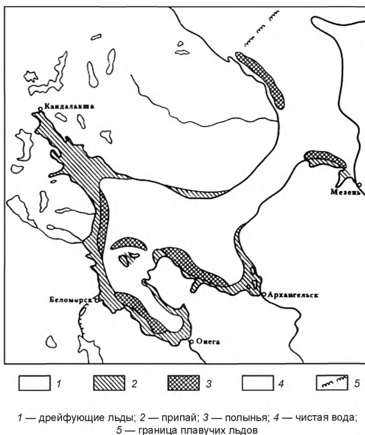
Рисунок В.15 — Ледяной покров в Белом море зимой
