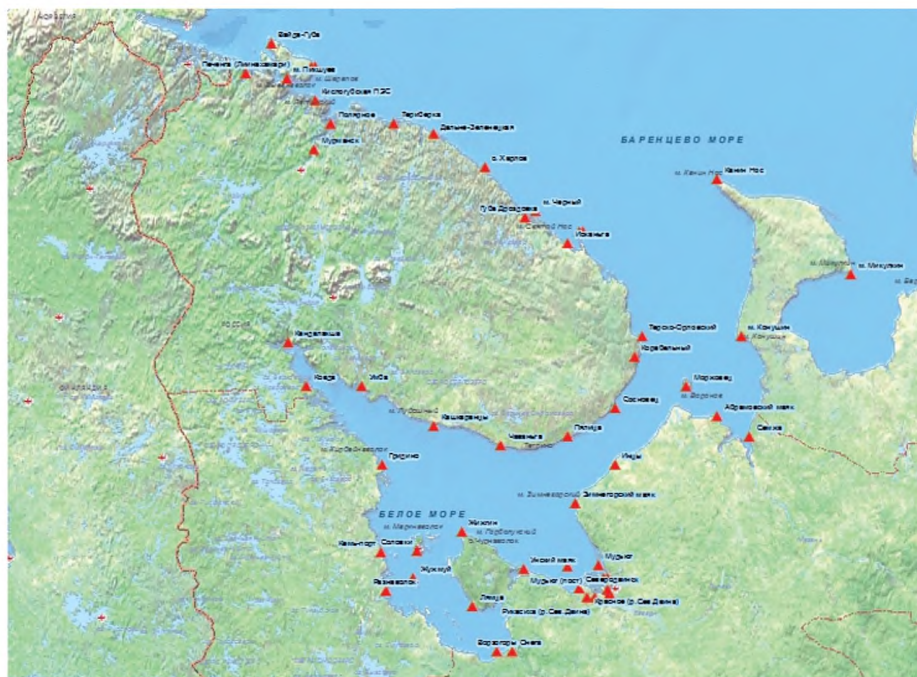
Рисунок В.13 — Схемы расположения морских гидрометстанций и постов Белого моря
