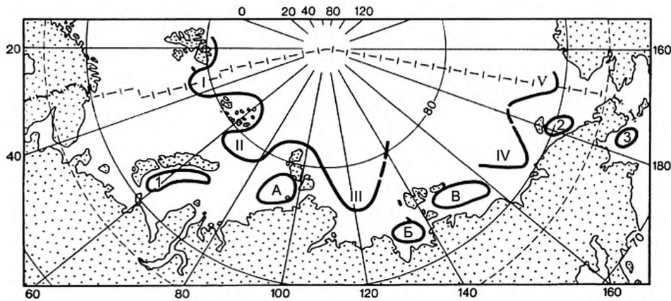
Отроги океанических массивов: I — Шпицбергенский; II — Карский; III — Таймырский; IV — Аионский; V — Чукотский. Локальные массивы дрейфующих льдов: 1 — Новоземельский, 2 — Врангелевский, 3 — Анадырский. Локальные массивы припайных льдов: А — Североземельский, Б — Янский, В — Новосибирский
