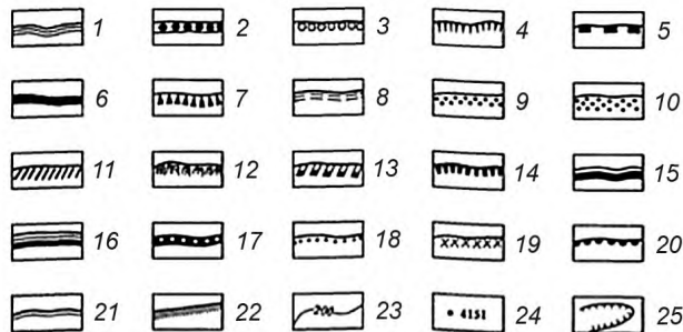
Рисунок В.8 — Типы берегов и рельеф дна Азовского моря
