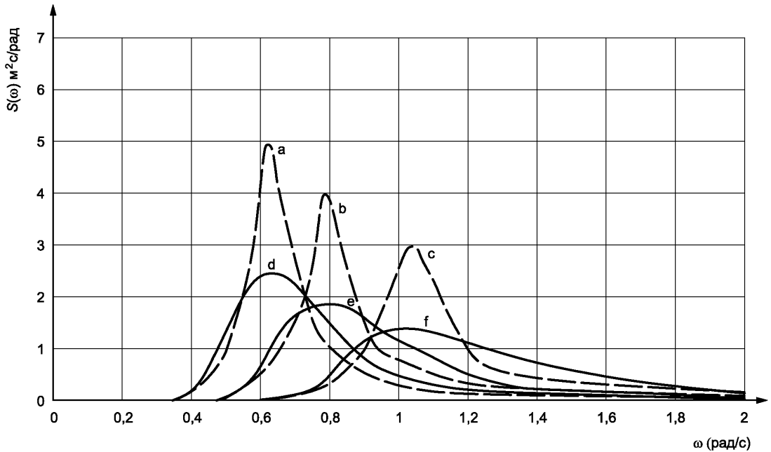
a — Спектр JONSWAP, T_p = 10 с; b — Спектр JONSWAP, T_p = 8 с; c — Спектр JONSWAP, T_p = 6 с; d — Спектр Пирсона-Московица, T_p = 10 с; e — Спектр Пирсона-Московица, T_p = 8 с; f — Спектр Пирсона-Московица, T_p = 6 с
