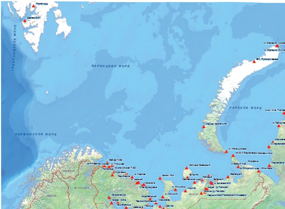
Рисунок В.21 — Схемы расположения морских гидрометеорологических станций и постов море Лаптевых
