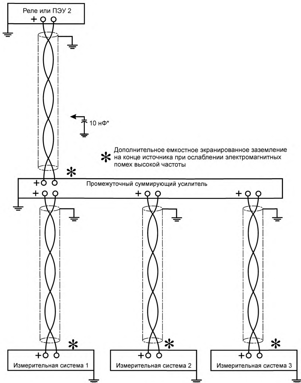
Рисунок 4 — Несколько измерительных систем и промежуточное устройство
