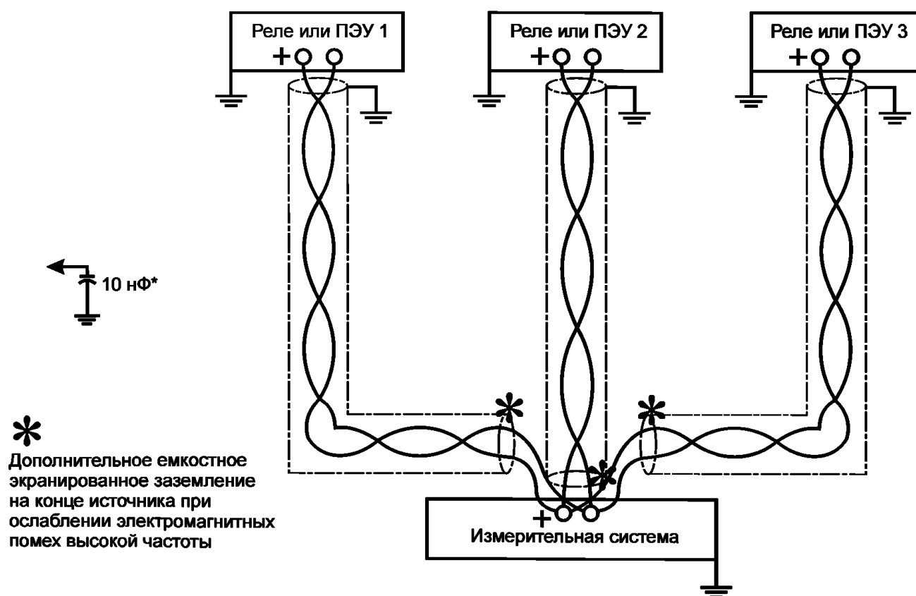
Рисунок 3 — Одна измерительная система с несколькими входами реле
