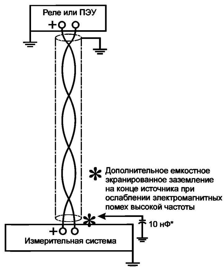
Рисунок 2 — Одна измерительная система и один вход реле
