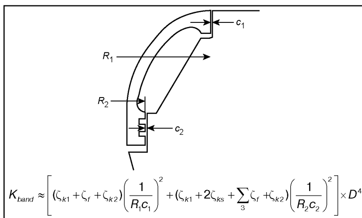
Рисунок Е.2 — Примеры типичной конструкции уплотнения рабочего колеса (сторона обода)
