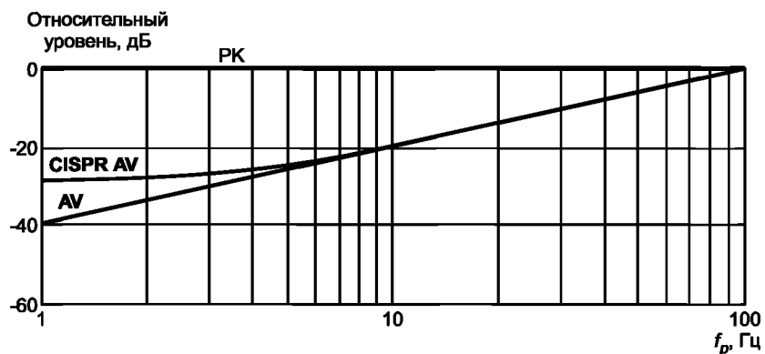
Рисунок С.2 — Весовая функция импульса 10 мс при детектировании пиковым детектором «PK», детектором средних значений при учете пиковых значений «CISPR AV» и детектором средних значений без учета пиковых значений «AV» для постоянной времени прибора 100 мс
