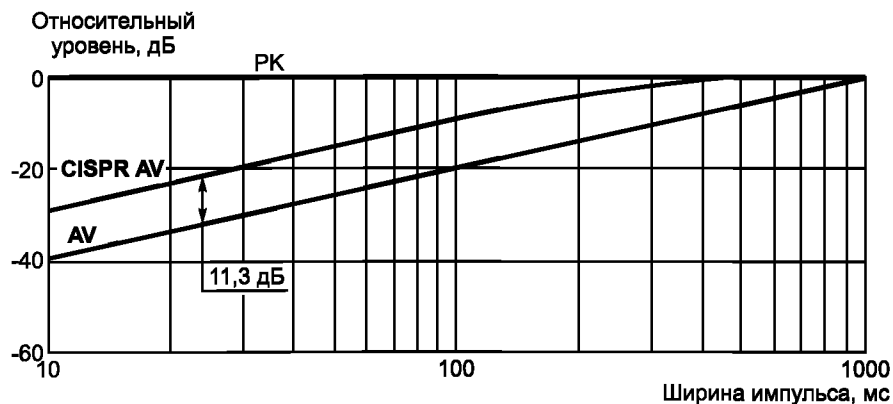
Рисунок С.4 — Пример весовых функций (импульс 1 Гц) при детектировании пиковым детектором «PK» и детектором средних значений «AV» относительно ширины импульсов для постоянной времени прибора 100 мс
