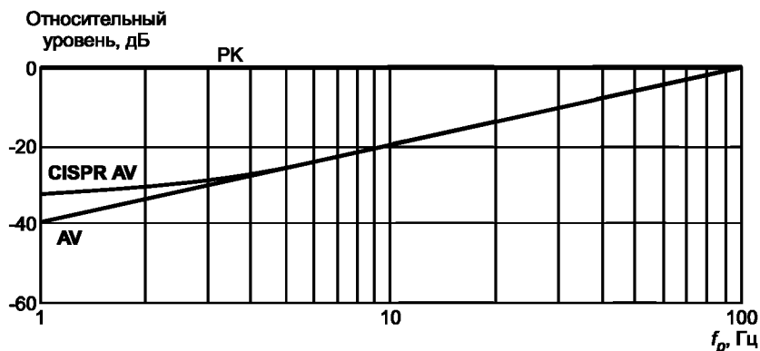
Рисунок С.1 — Весовая функция импульса 10 мс при детектировании пиковым детектором «PK», детектором средних значений при учете пиковых значений «CISPR AV» и детектором средних значений без учета пиковых значений «AV» для постоянной времени прибора 160 мс
