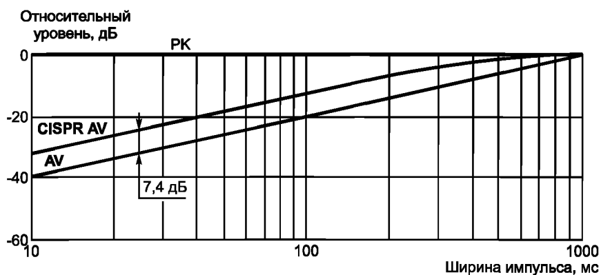
Рисунок С.3 — Пример весовых функций (импульс 1 Гц) при детектировании пиковым детектором «PK» и детектором средних значений «AV» относительно ширины импульсов для постоянной времени прибора 160 мс
