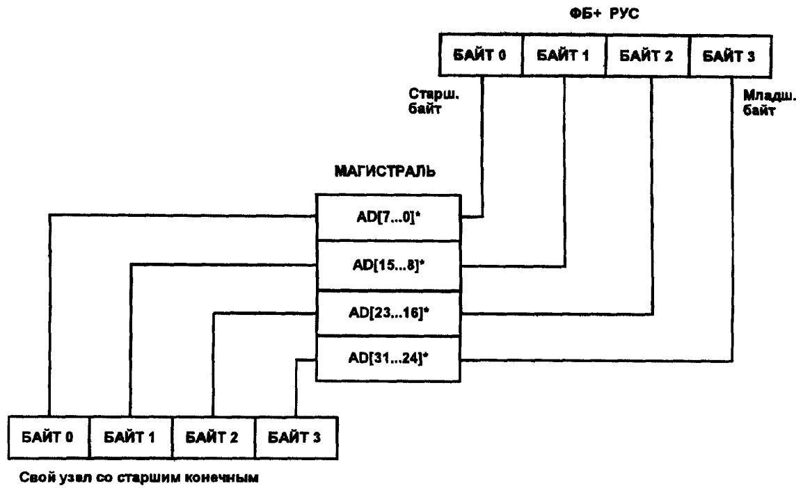
Рисунок 3—3(а) — Расположение байтов РУСа
