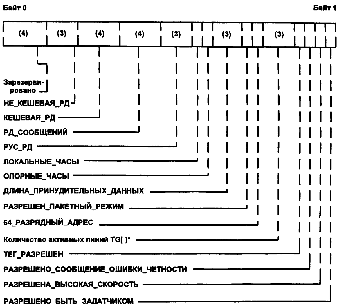
Рисунок 3–23 — Формат регистра ЛОГИЧЕСКОГО_УПРАВЛЕНИЯ_МОДУЛЯ
