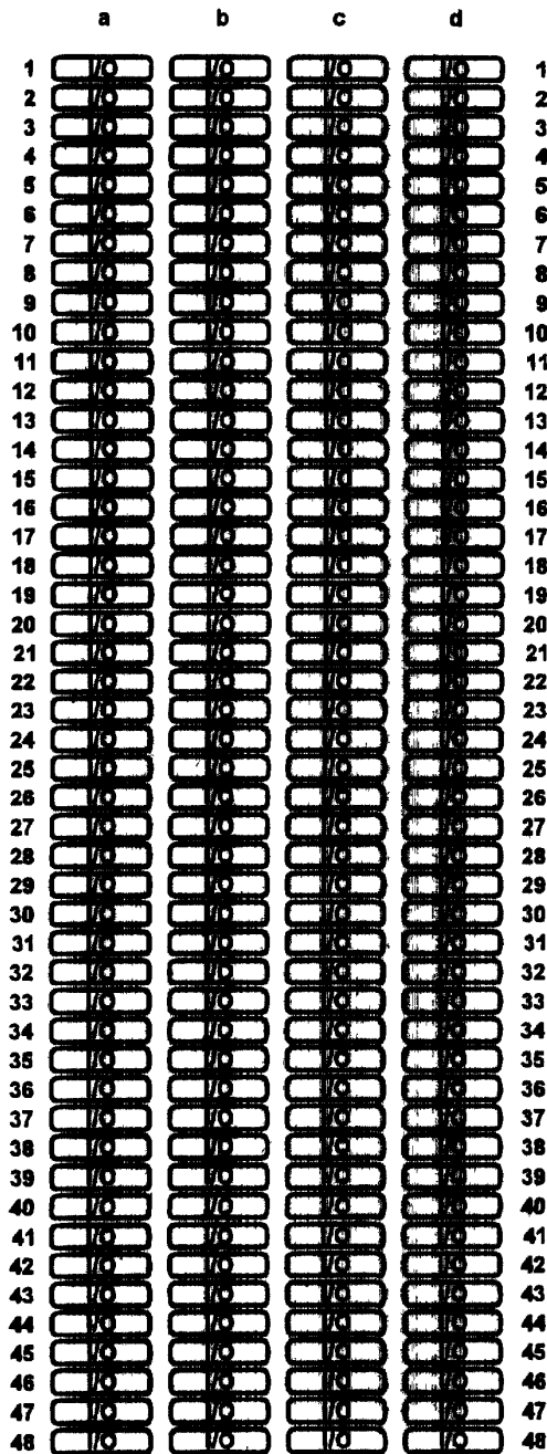
Рисунок 6—16 — Распределение контактов разъема Е для 192 ввода/вывода
