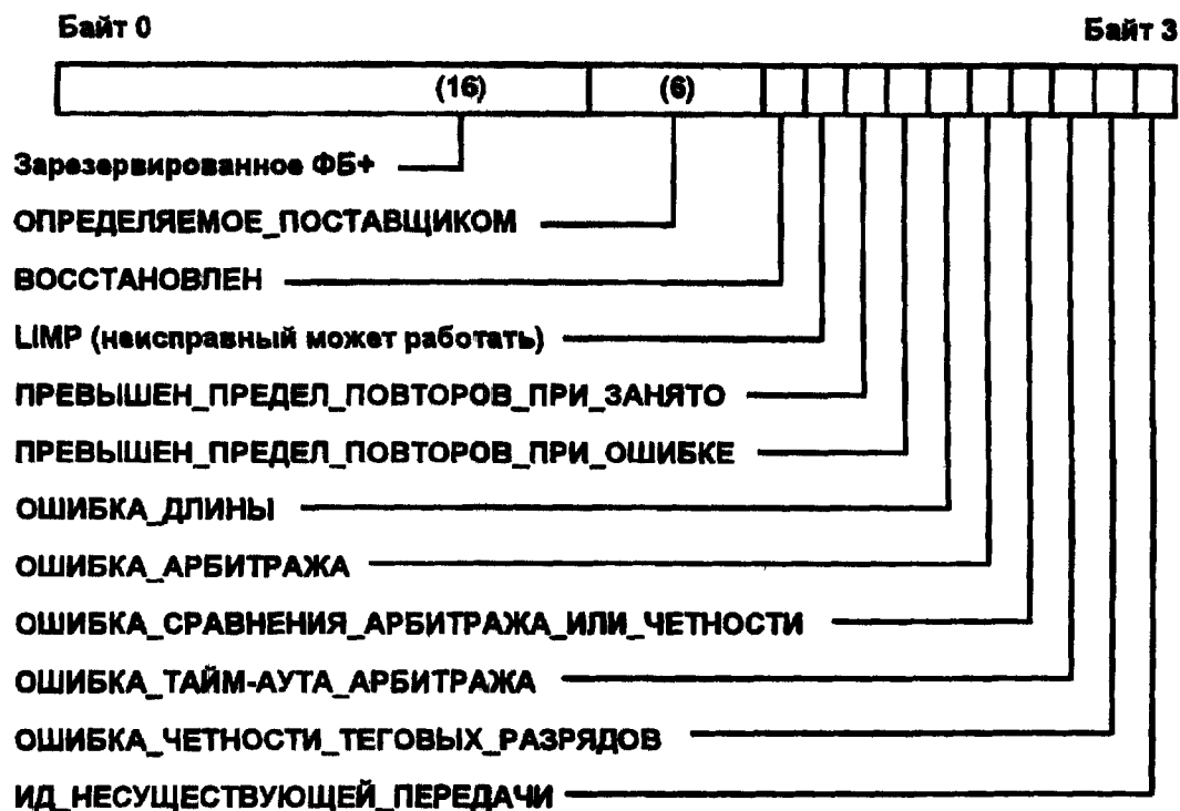
Рисунок 3—20 — Формат данных РУСа ОШИБКА_МЛАДШ.
