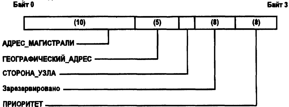
Рисунок 3—6 — Формат данных РУСа ИДЕНТИФИКАТОРЫ_УЗЛА
