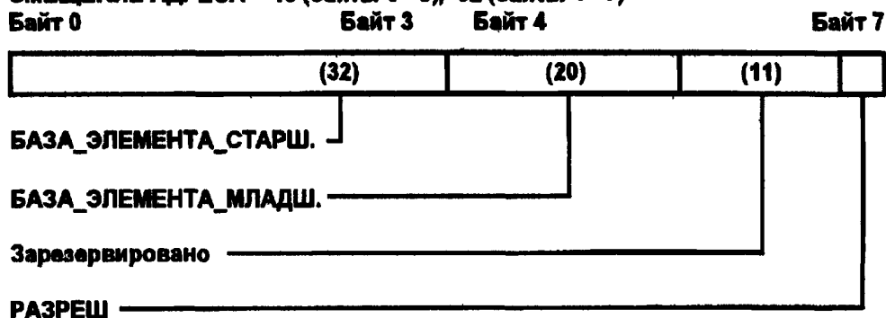
Рисунок 3—14 — Формат данных РУСа БАЗА_ЭЛЕМЕНТОВ
