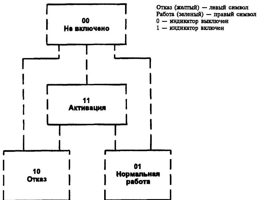
Рисунок 7—10 — Диаграмма состояний модуля
