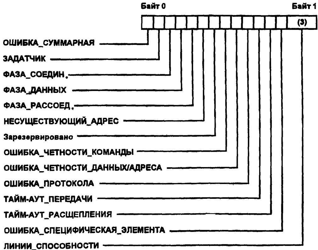
Рисунок 3—19(а) — Формат данных РУСа ОШИБКА_СТАРШ (старшая половина)
