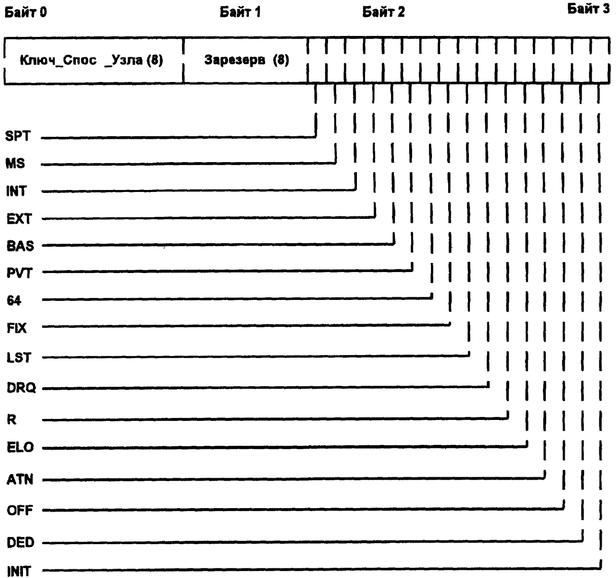
Рисунок 3—33 — Формат Входа СПОСОБНОСТИ_УЗЛА
