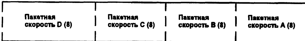
Рисунок 3—31 — Формат РУС СКОРОСТЬ_ПАКЕТА
