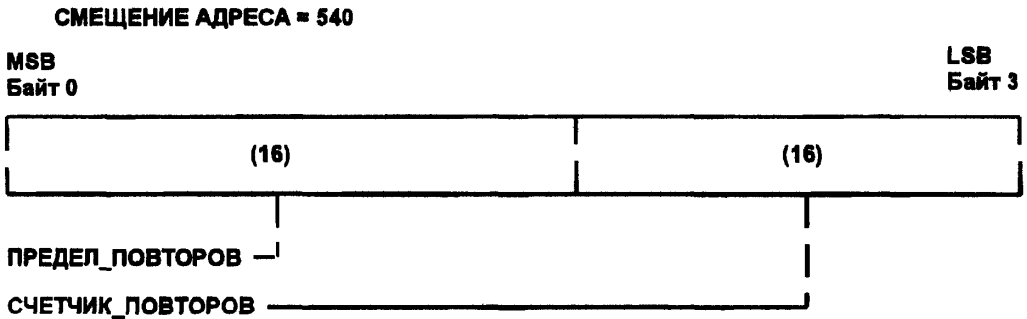
Рисунок 3—24 — Регистр СЧЕТЧИК_ПОВТОРОВ_ПРИ_ЗАНЯТОСТИ
