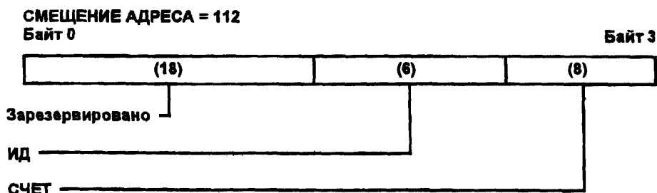
Рисунок 3—18 — Формат данных РУСа СТРОБ_ЧАСОВ
