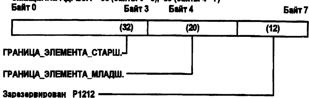
Рисунок 3—15 — Формат данных РУСа ГРАНИЦА_ЭЛЕМЕНТОВ
