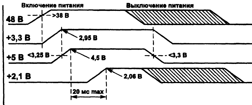
Рисунок 7—2 — Временная последовательность напряжений питания Профиля Б
