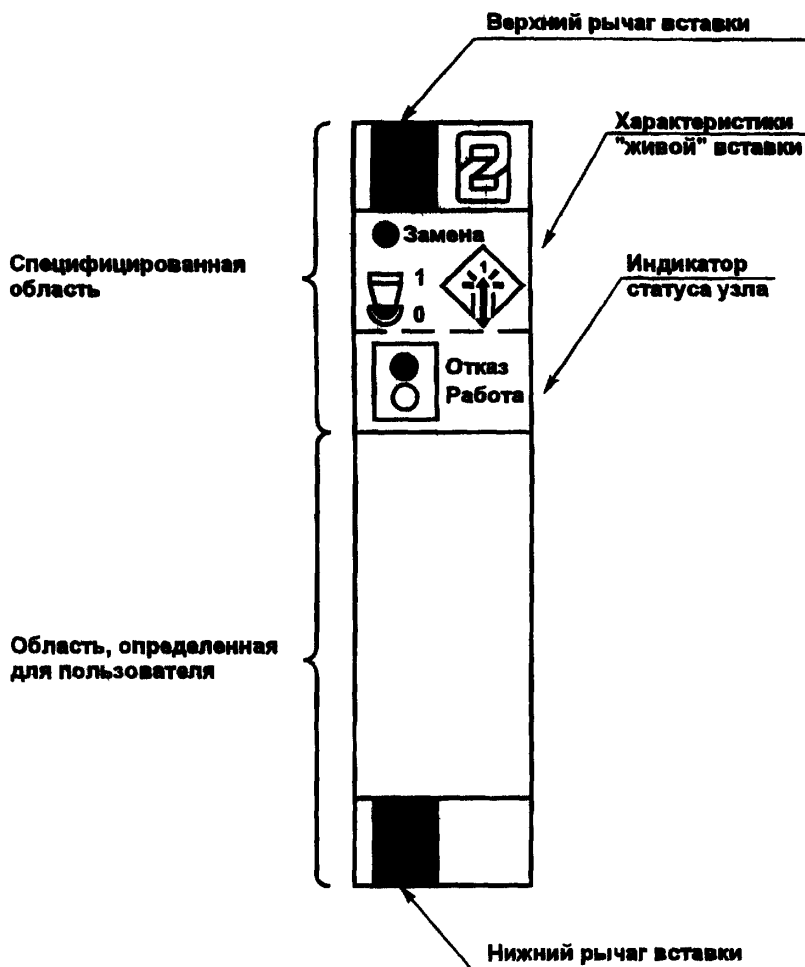
Рисунок 6—9 — Организация передней панели профиля А
