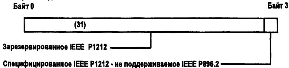
Рисунок 3—7 — Формат данных РУСа СТАРТ_СБРОСА
