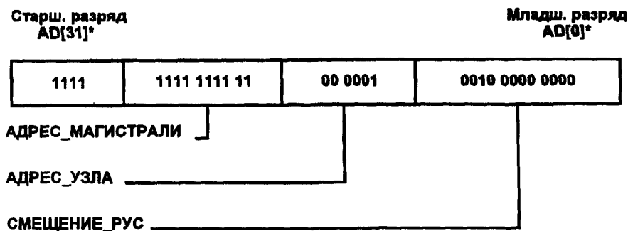
Рисунок 3—2(в) — Адресация 32-разрядных РУС
