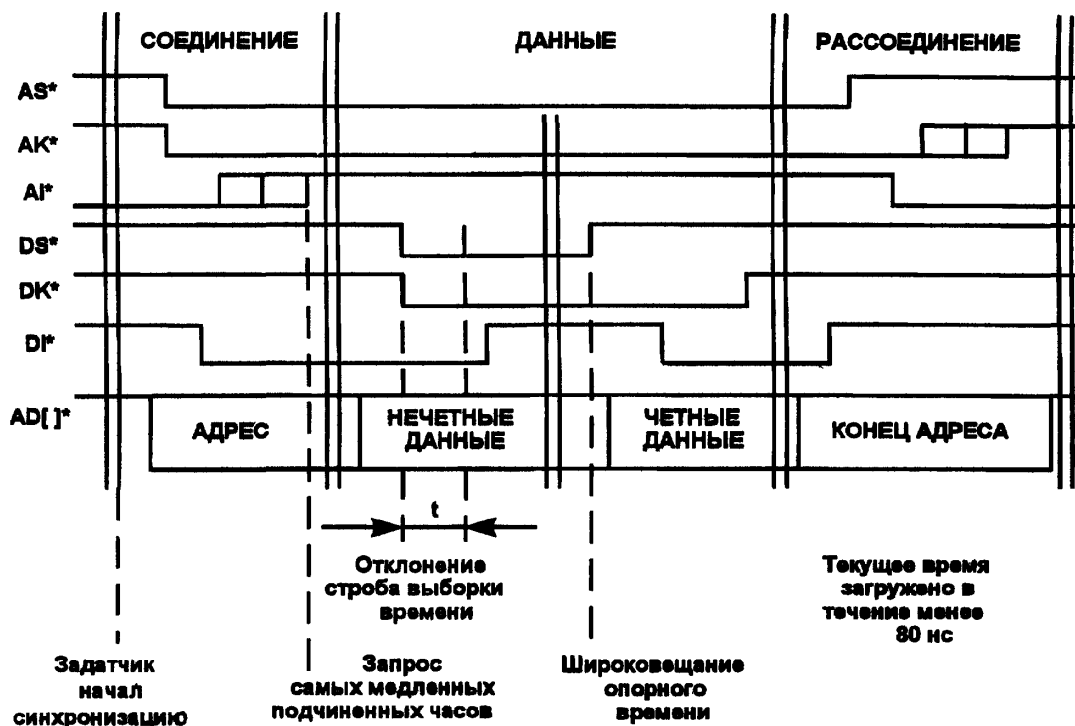
Рисунок 3—4 — Синхронизация часов
