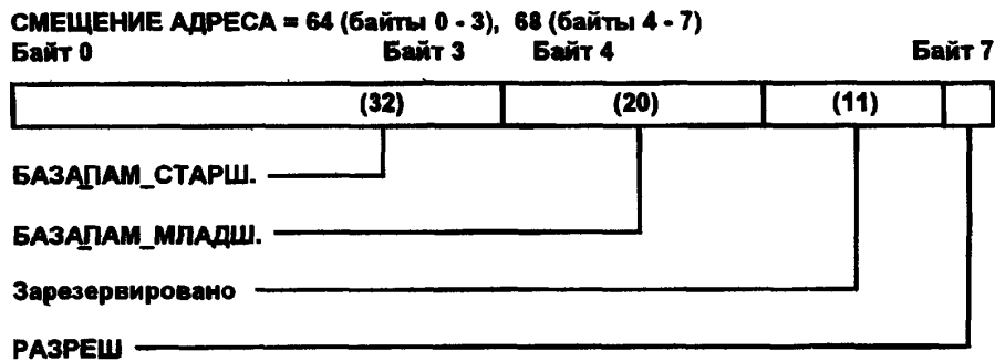
Рисунок 3—16 — Формат данных РУС БАЗА_ПАМЯТИ
