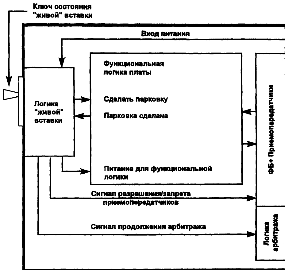
Рисунок 4—2 — Функциональное строение модуля с «живой» вставкой
