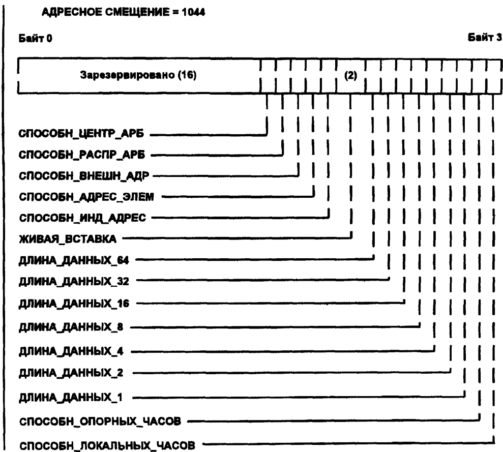
Рисунок 3—29 — Формат РУС ВНЕШНИЕ_СПОСОБНОСТИ_УЗЛА
