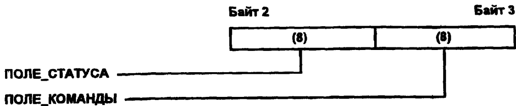
Рисунок 3—19(б) — Формат данных РУСа ОШИБКА_СТАРШ (младшая половина)
