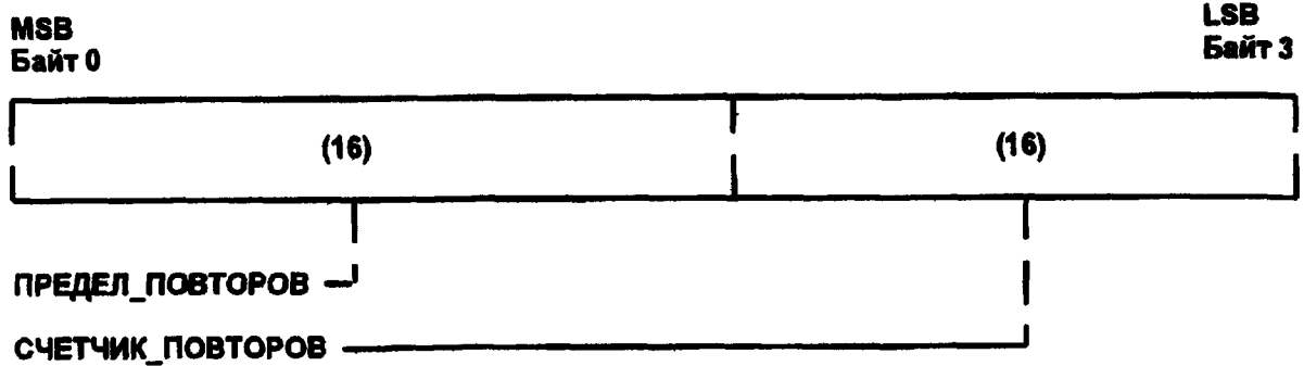
Рисунок 3—26 — Регистр СЧЕТЧИК_ПОВТОРОВ_ПРИ_ОШИБКЕ
