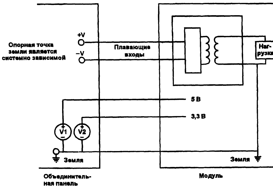
Рисунок 7—1 — Шины питания Профиля Б
