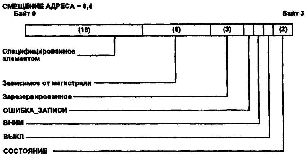
Рисунок 3—5 — Поля в РУСх ОЧИСТКА_СОСТОЯНИЯ и УСТАНОВКА_СОСТОЯНИЯ, используемые в ФБ+.
