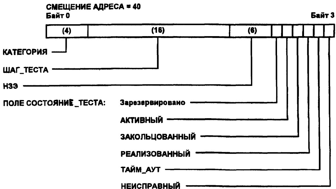
Рисунок 3—13 — Формат данных РУСа СТАТУС_ТЕСТА
