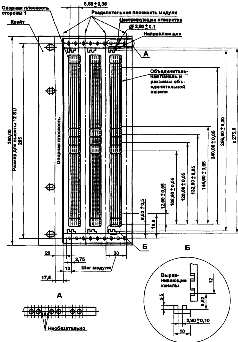
Рисунок 6-2 — Вид соединения Крейт/Объединительная плата
