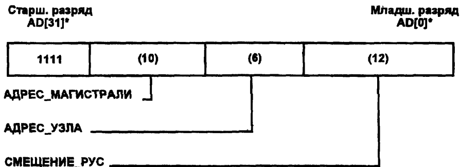
Рисунок 3—2(б) — Адресация 32-разрядных РУС
