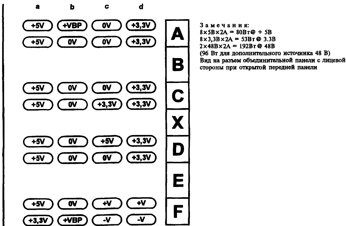
Рисунок 7—16 — Распределение контактов питания для разъемов профиля Б
