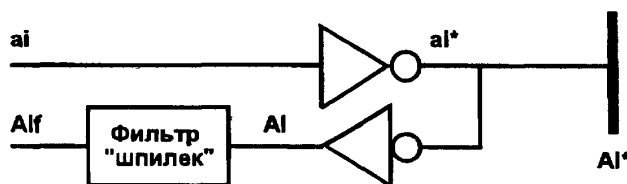
Рисунок 2.1 — Соглашения о сигналах
