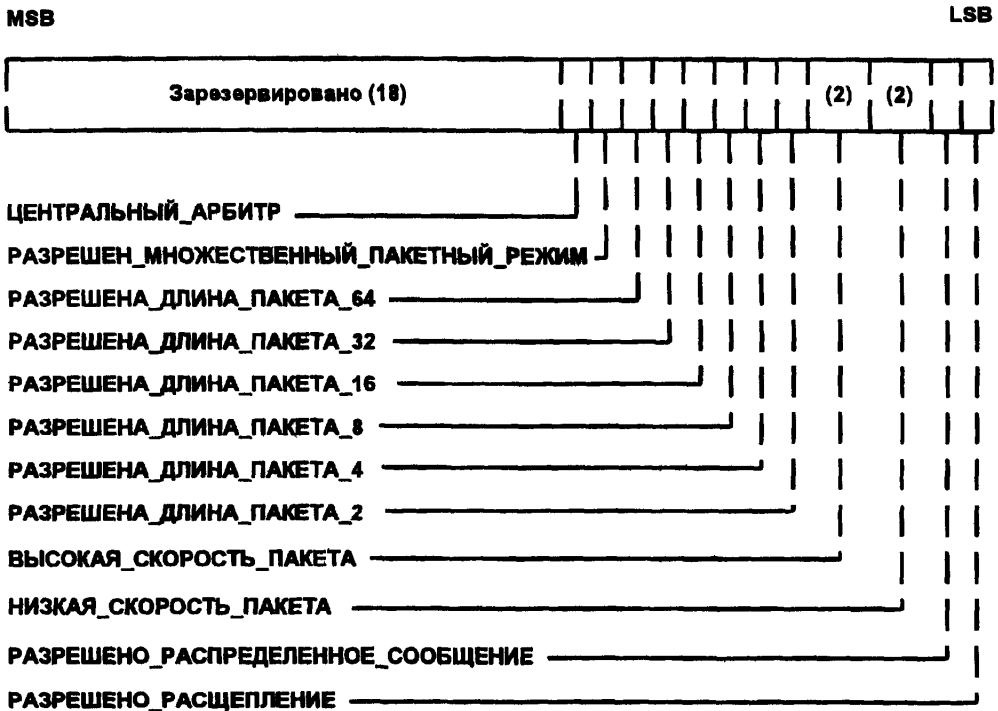
Рисунок 3—22 — Формат регистра ОБЩЕГО_ЛОГИЧЕСКОГО_УПРАВЛЕНИЯ
