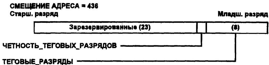
Рисунок 3—21 — Формат данных РУСа УДЕРЖАНИЕ_ТЕГОВ
