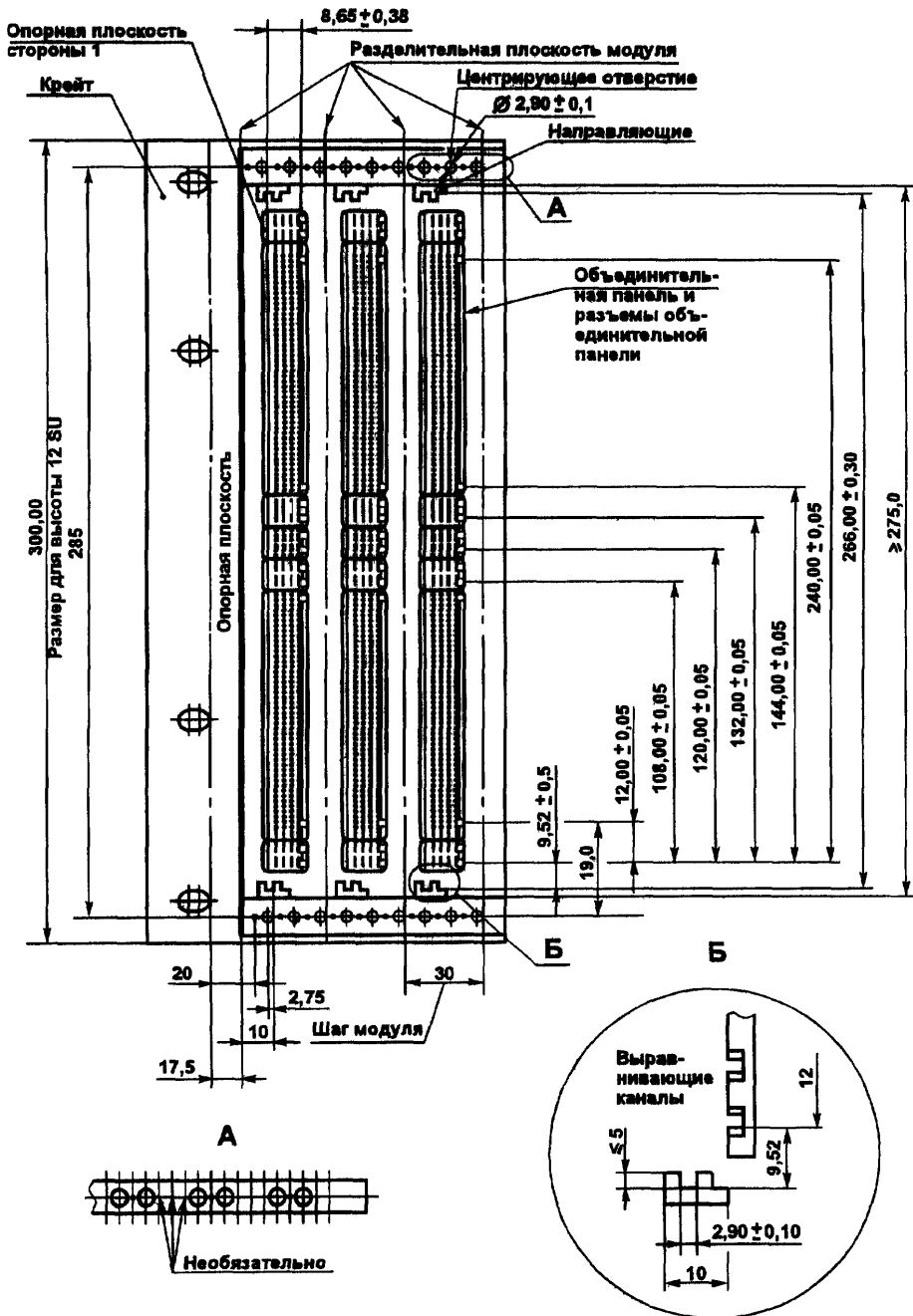
Рисунок 7-3 — X-Y вид соединения крейта и модуля
