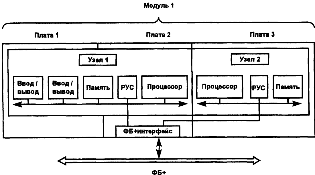
Рисунок 3—1 — ФБ+ платы, модули, узлы
