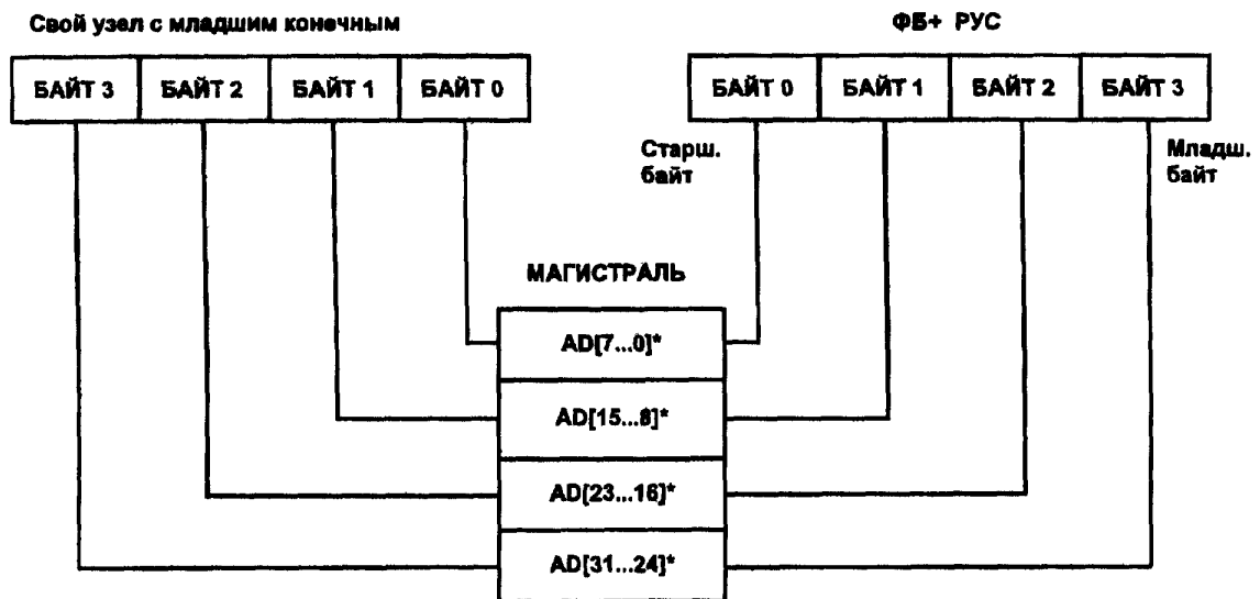
Рисунок 3—3(б) — Расположение байтов РУСа
