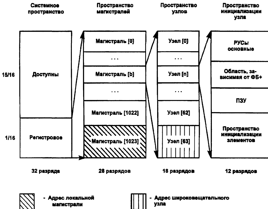
Рисунок 3—2(а) — Адресация 32-разрядных РУС
