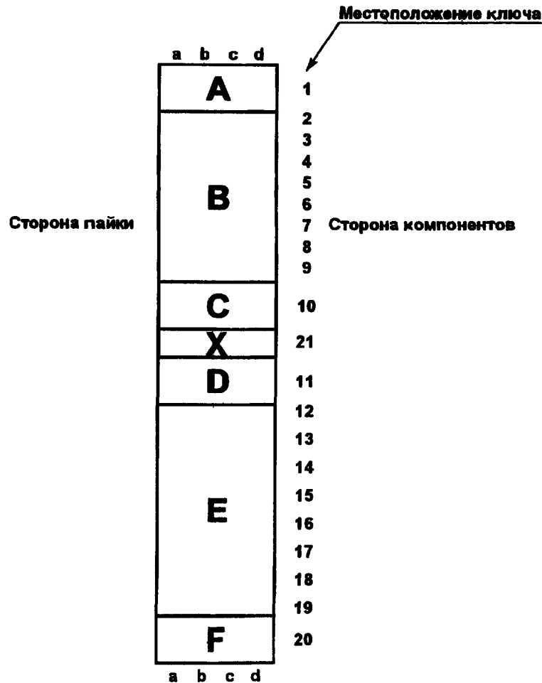
Рисунок 6—13 — Соглашения по наименованию разъемов
