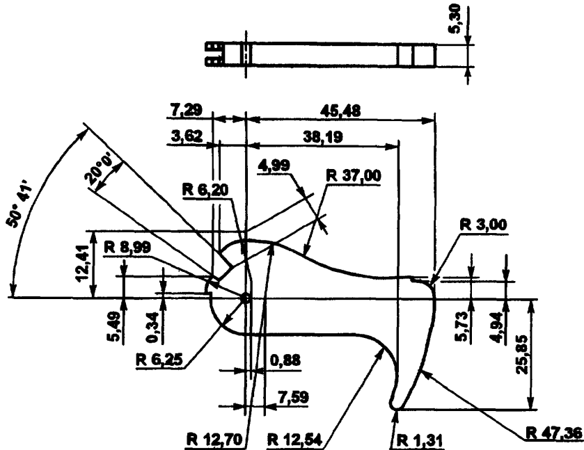
Рисунок 7—7 — рекомендуемый для Профиля Б рычаг вставки/вынимания
