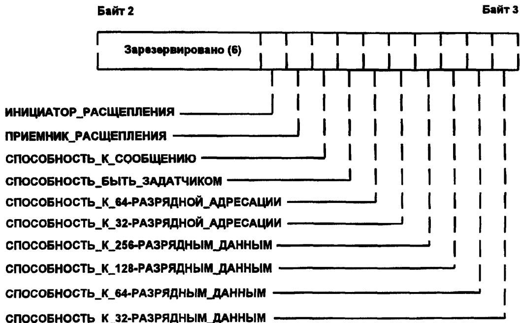
Рисунок 3—28(б) — ЛОГИЧЕСКАЯ СПОСОБНОСТЬ МОДУЛЯ (Младшая половина)
