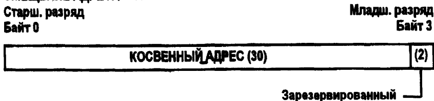
Рисунок 3—8 — Формат данных внутреннего РУСа КОСВЕННЫЙ_АДРЕС
