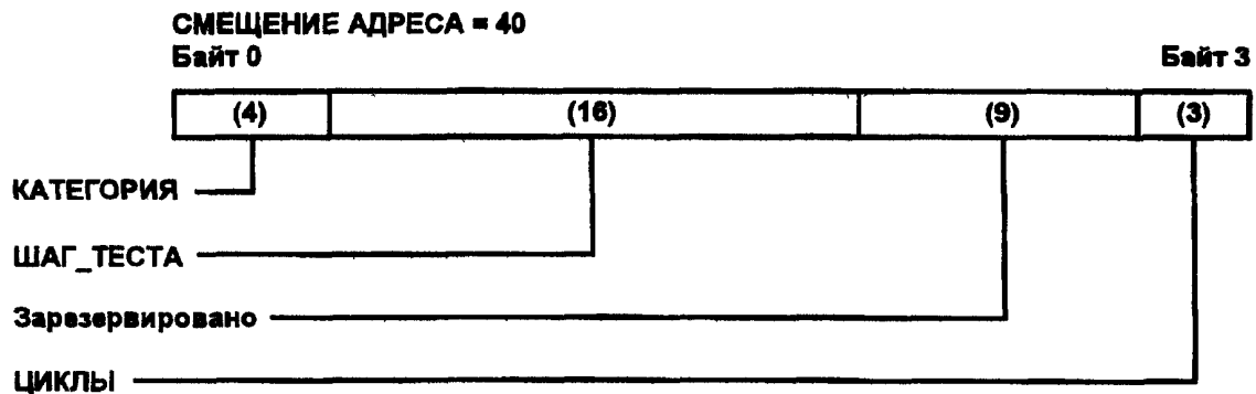
Рисунок 3—12 — Формат данных РУС СТАРТ_ТЕСТА
