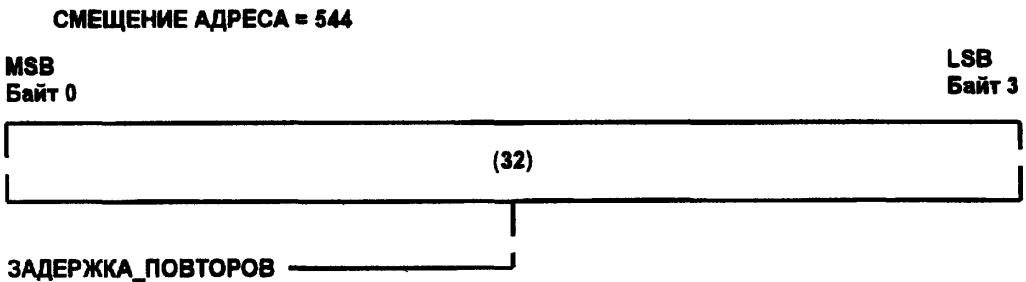
Рисунок 3—25 — Регистр ЗАДЕРЖКА_ПОВТОРОВ_ПРИ_ЗАНЯТОСТИ
