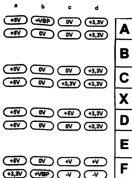
Рисунок 6—18 — Распределение контактов питания для разъемов профиля А
