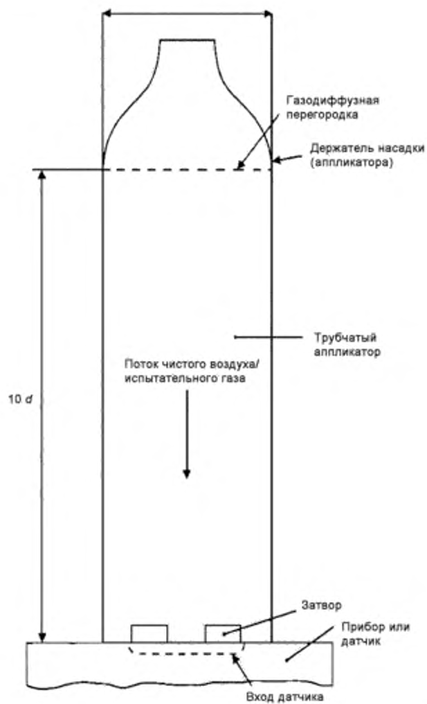
Рисунок В.4 – Примерная схема апликатора и входного отверстия датчика при подаче испытательного газа или чистого воздуха
