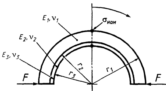
Рисунок А.1 — Система вкладыша
