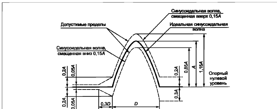
Рисунок 2 – Форма полусинусоидального импульса ускорения и его допустимые пределы
