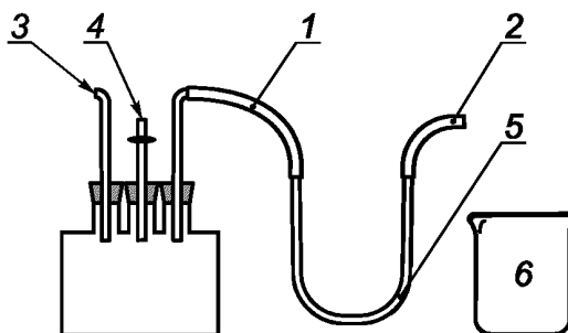
1 — трубка 1; 2 — трубка 2; 3 — водоструйный насос; 4 — запорный кран; 5 — стеклоянная колонка; 6 — диметилдихлорсилан и толуол
