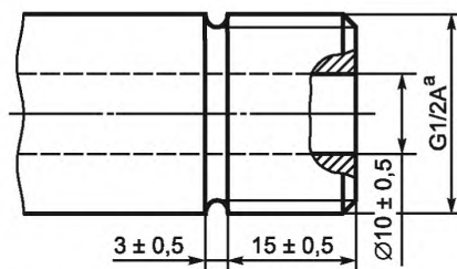
a Трубная резьба по ISO 228-1 G1/2A.
