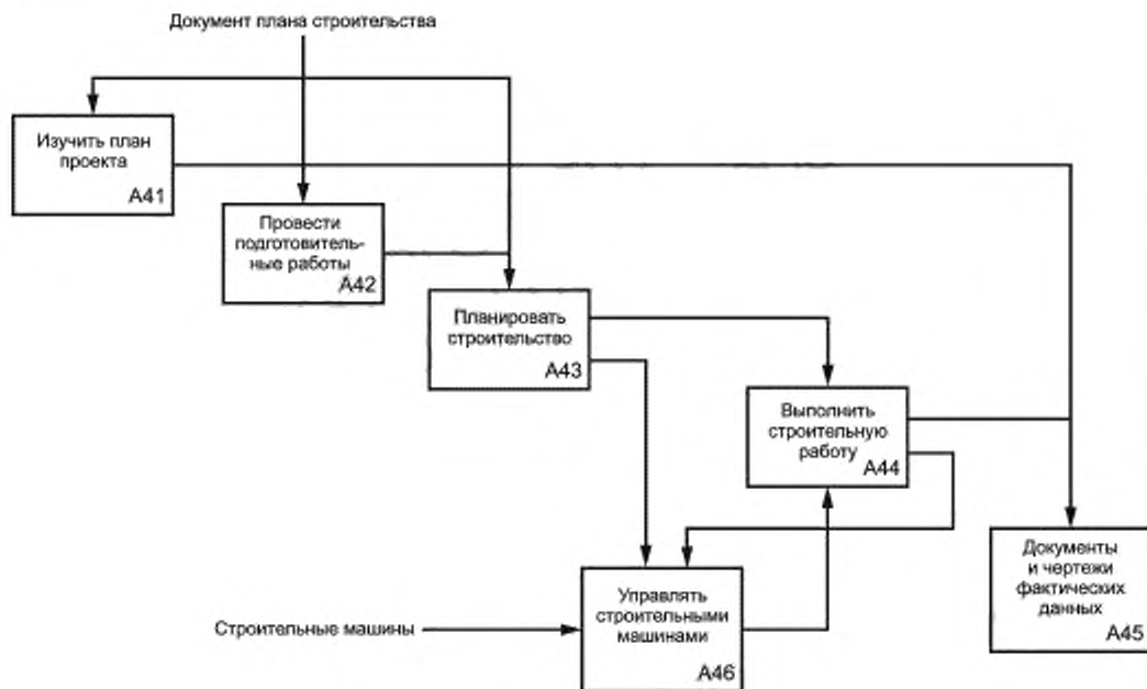
Рисунок E.2 — Рабочий процесс этапа строительства (IDEF0)
