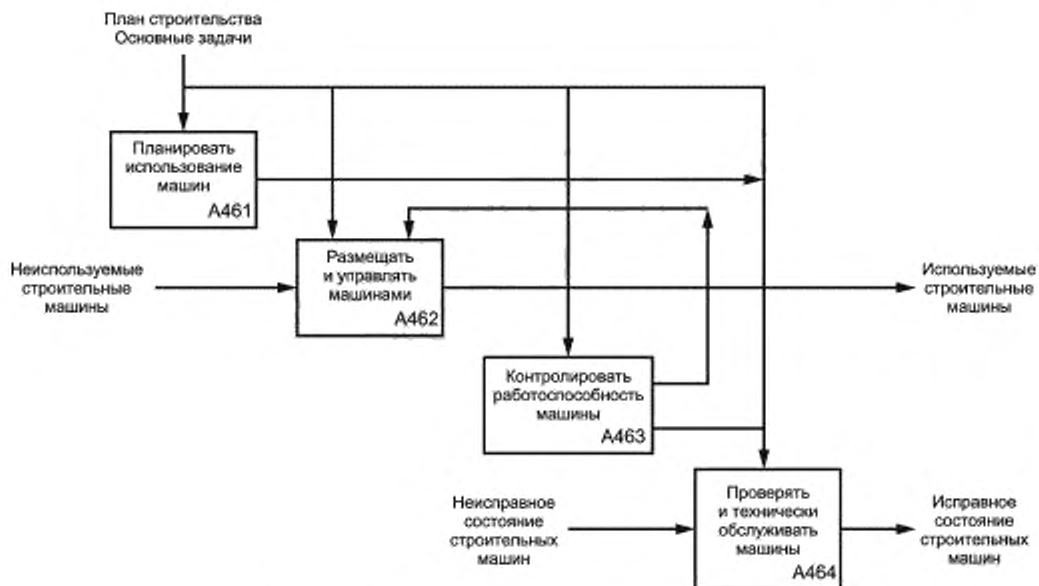
Рисунок Е.4 — Процесс управления машиной (IDEF0)
