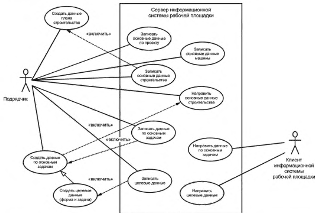
Рисунок D.3 — Диаграмма варианта использования. Услуга по представлению данных по основным задачам и целевым данным
