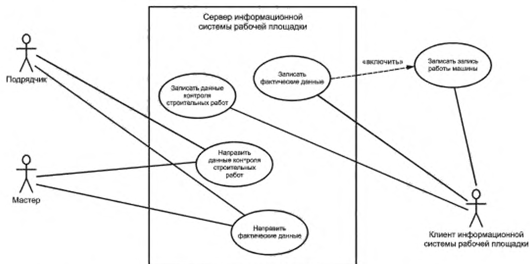
Рисунок D.6 — Диаграмма варианта использования. Услуга по представлению достигнутых результатов
