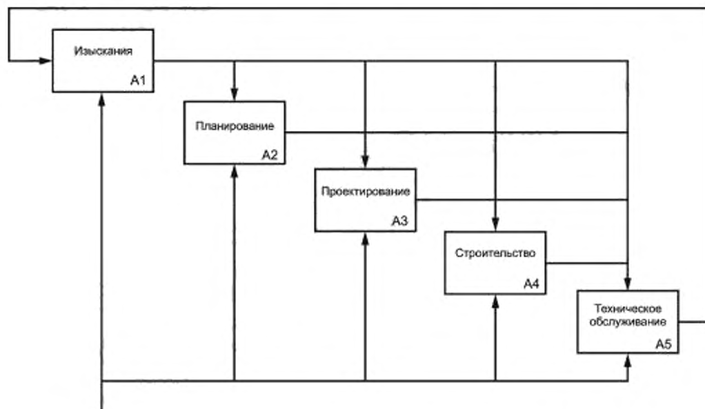
Рисунок Е.1 — Жизненный цикл строительного проекта (IDEF0)
