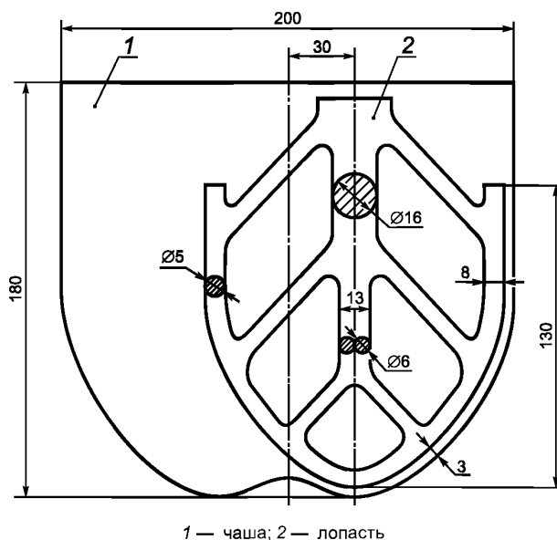
1 — чаша; 2 — лопасть
