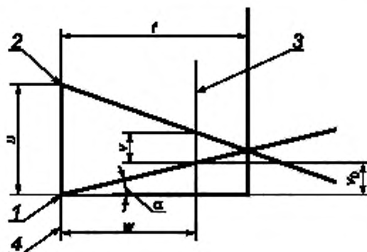
f — луч 1; 2 — луч 2; 3 — измерительная плоскость; 4 — испытуемый светофильтр; f — фокусное расстояние светофильтра; u — расстояние между параллельными лучами 1 и 2; v — расстояние между точками пересечения преломленными лучами 1 и 2 плоскости измерения; w — расстояние между испытуемым светофильтром и измерительной плоскостью; \alpha — угол отклонения осевого луча 1, v_f — отклонение осевого луча от оптической оси в плоскости измерения
