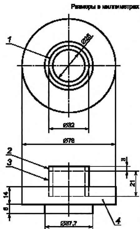
1 — силиконовая прокладка; 2 — силиконовая прокладка; 3 — опорная труба; 4 — испытательный блок
