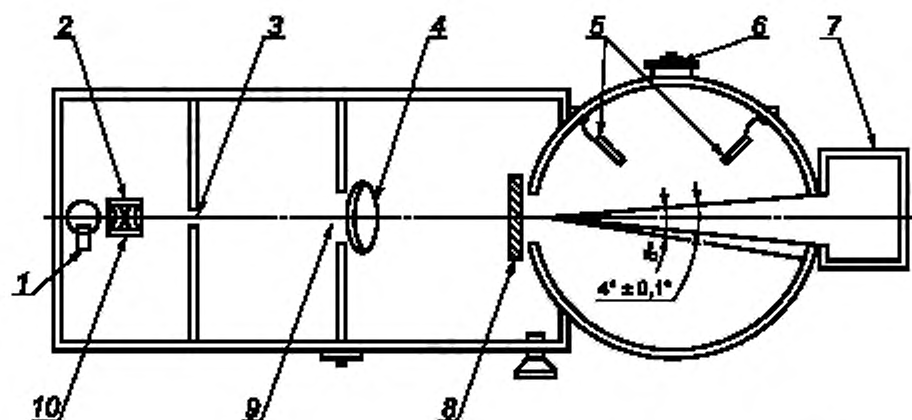
1 — источник излучения; 2 — конденсор; 3 — входное окно; 4 — линза; 5 — отражатели; 6 — фотоэлемент; 7 — световая ловушка; 8 — испытуемый образец; 9 — диафрагма, 10 — светофильтр
