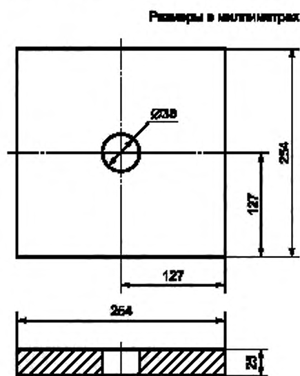
Рисунок 17 — Опора образца
