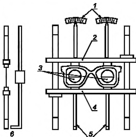
1 — шкалы; 2 — верхняя регистровая рейка; 3 — поляризаторы с разделенными полями; 4 — нижняя регистровая рейка; 5 — рычаги вращения поляризаторов; 6 — вид сбоку
