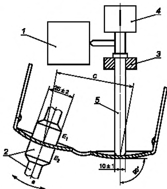
1 — измерительное устройство; 2 — кольцевой зажим; 3 — движущееся кольцо; 4 — направление и точка приложения силы (максимум 5 Н); 5 — прижимной стержень; E_1 , E_2 — контактные поверхности; a — регулировка
