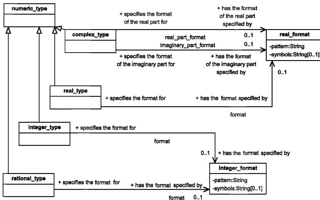
Рисунок 5 — Диаграмма класса UML для области числовых типов
