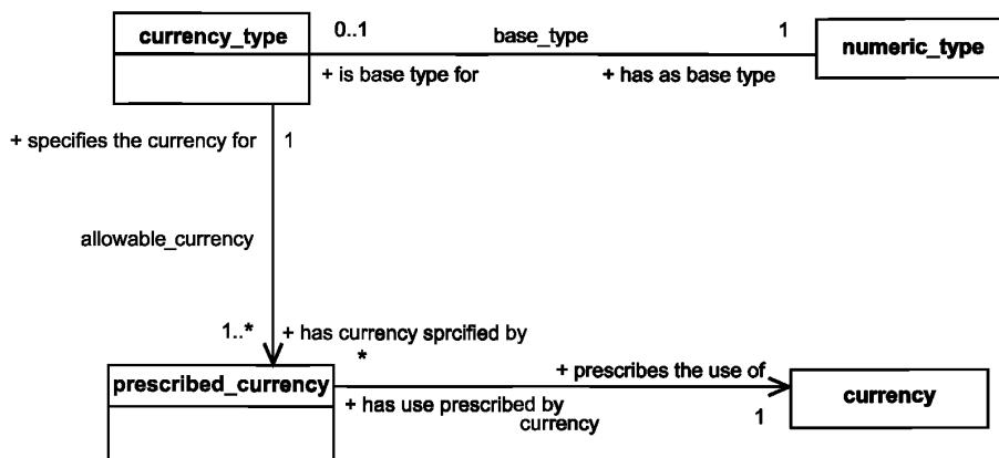
Рисунок 10 — Диаграмма класса UML для типа денежных единиц
