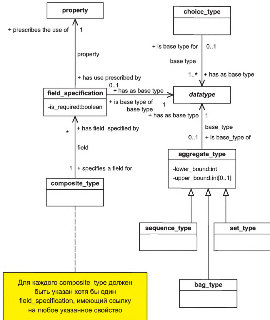
Рисунок 11 — Диаграмма класса UML для сложного типа
