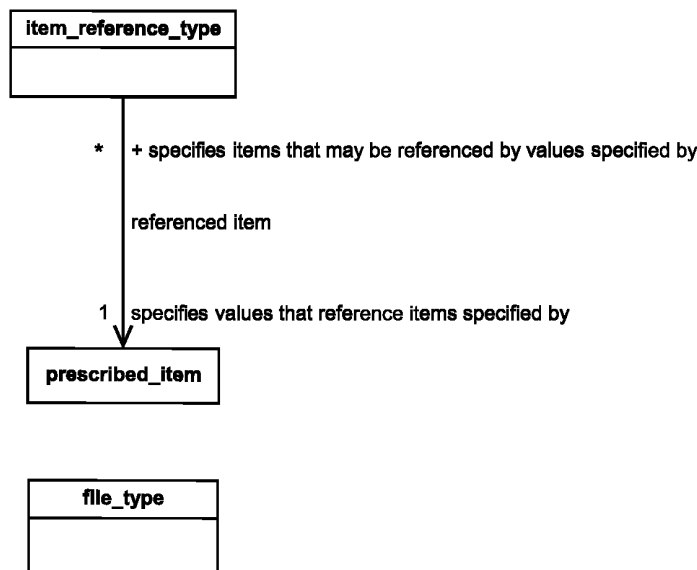
Рисунок 12 — Диаграмма класса UML для элементов ссылочного типа
