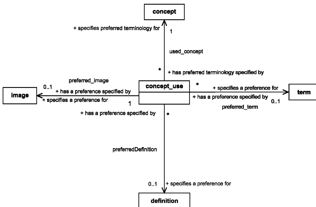
Рисунок 2 — Диаграмма класса UML, относящаяся к применению концепта
