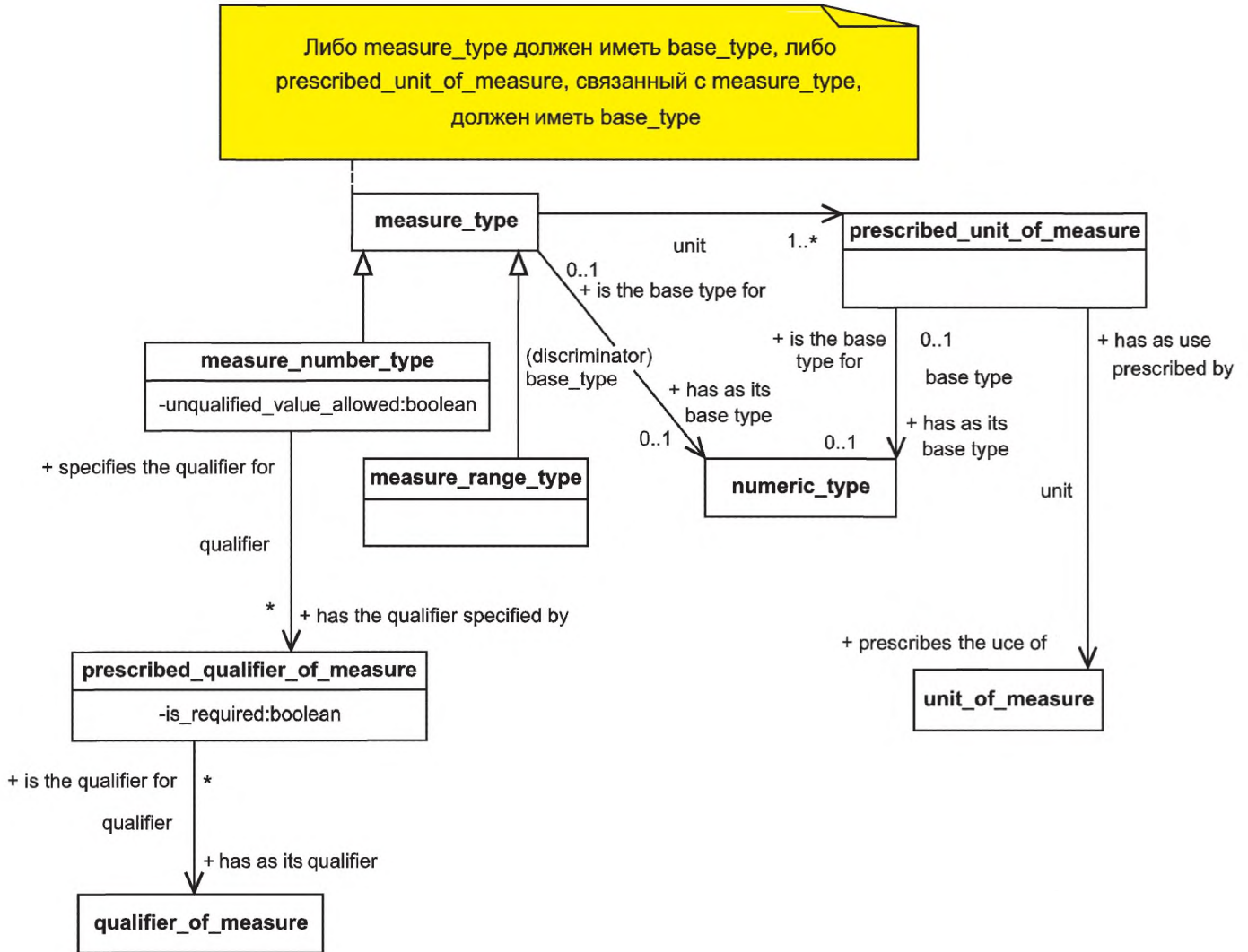
Рисунок 9 — Диаграмма класса UML для типов показателей
