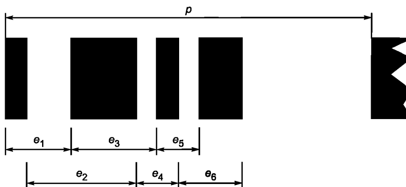
Рисунок J.1 — Размеры для декодирования
