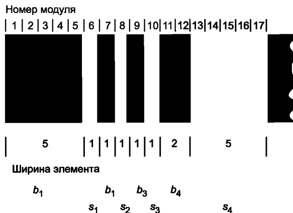
Рисунок 3 — Знак символа PDF417
