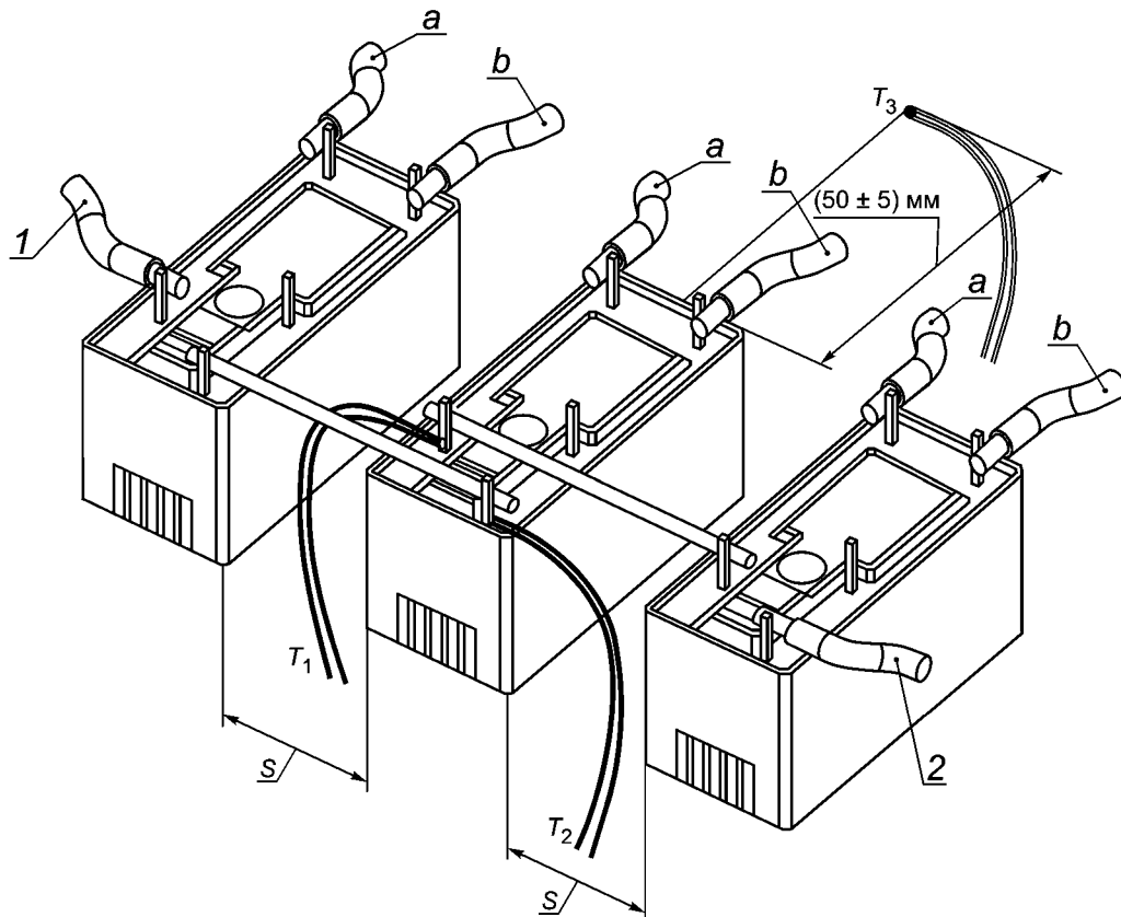
1, 2 — клеммы контактов; T_1 , T_2 , T_3 — термопары; a , b — клеммы катушек; S — расстояние монтажа
