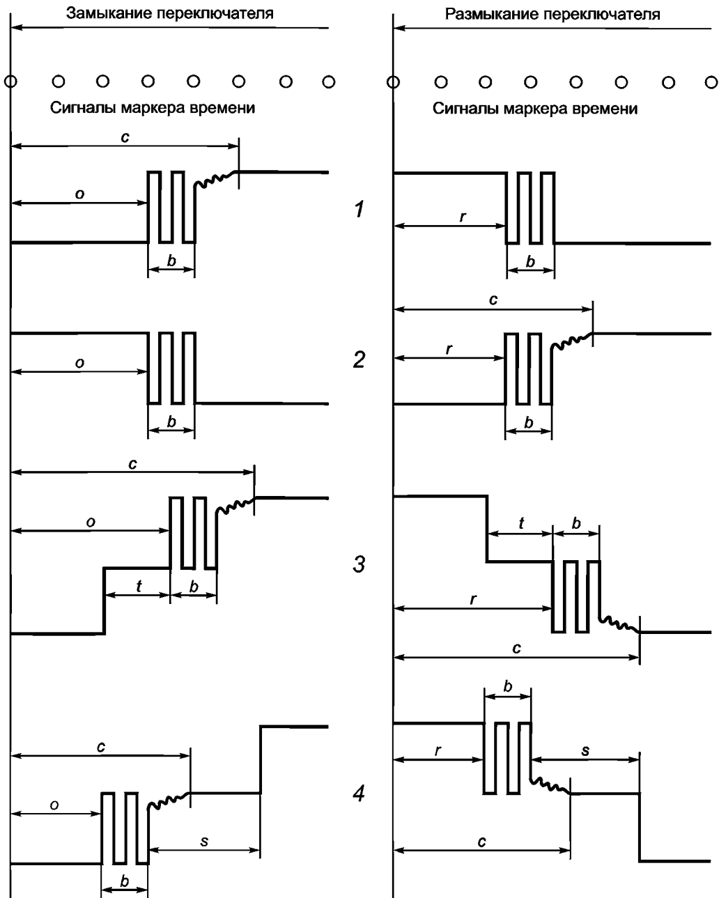
1 — замыкающий контакт; 2 — размыкающий контакт; 3 — размыкающий контакт перед замыканием; 4 — замыкающий контакт перед размыканием; o — время срабатывания реле; r — время возврата реле; b — время дребезга контактов; t — время перехода; s — время перекрытия контактов; c — время устойчивого замыкания
