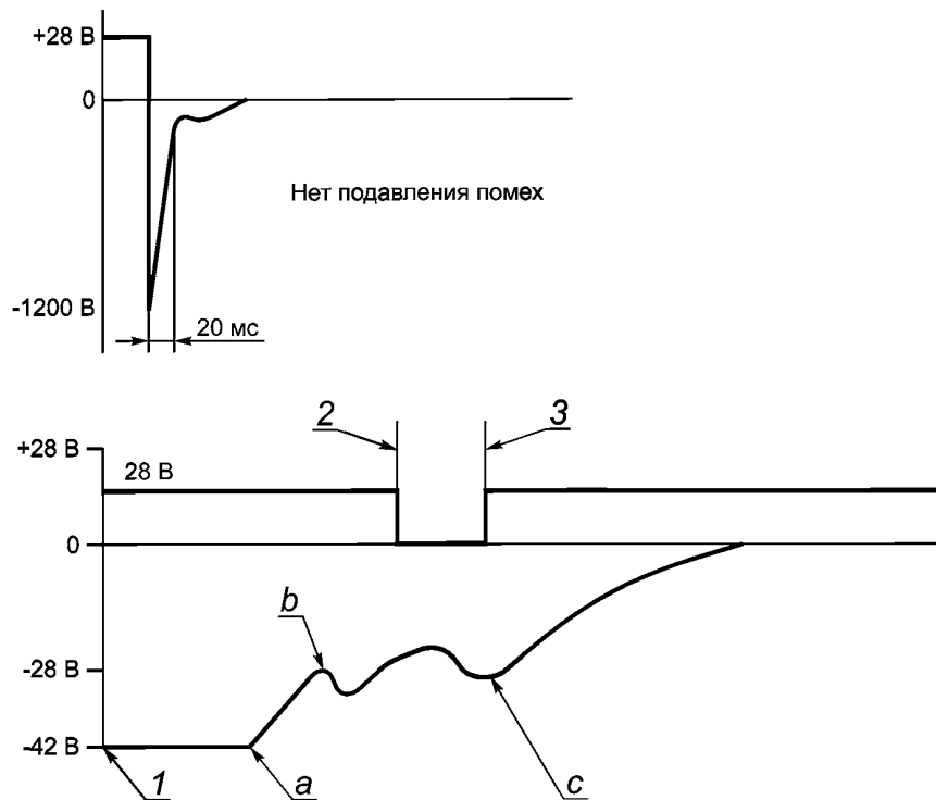
1 — контакт коммутационного реле разомкнут; 2 — контакт тестового реле разомкнут (размыкающий контакт); 3 — контакт тестового реле разомкнут (замыкающий контакт); a — срез вследствие использования компоненты подавления помех; b — начальное движение якоря; c — конечное движение якоря
