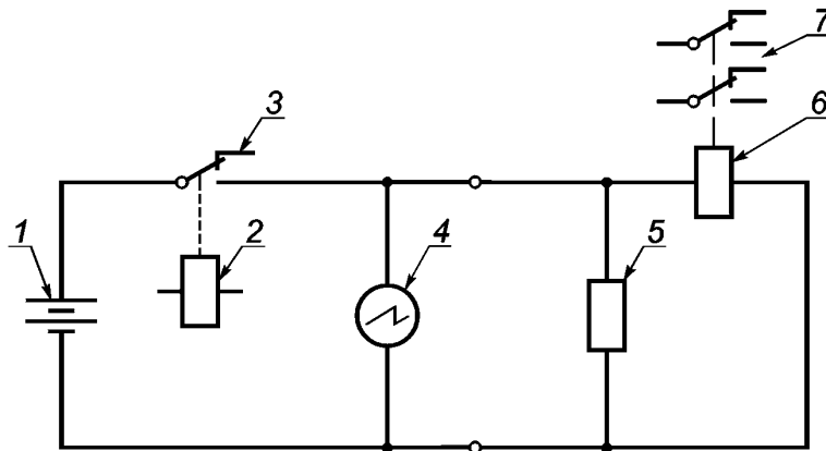
1 — подача возбуждения (низкий импеданс); 2 — катушка индуктивности коммутационного реле; 3 — контакт коммутационного реле (без дребезга); 4 — мониторинг прибор (осциллограф); 5 — схема подавления помех; 6 — катушка индуктивности испытуемого реле; 7 — контакты испытуемого реле
