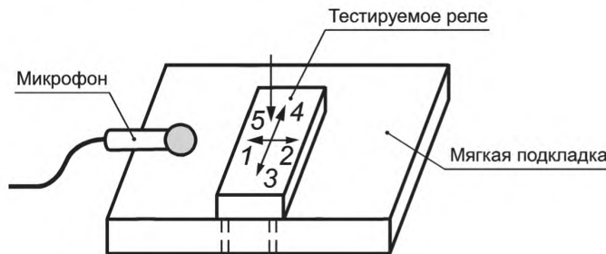
1, 2, 3, 4 и 5 — направления тестов
