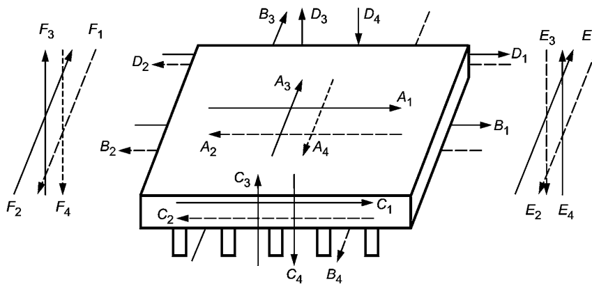
Направления тестового тока с A_1 по F_4
