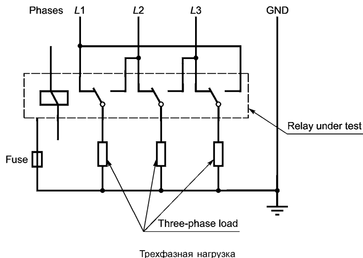
Рисунок 10 — Тестовая схема для переноса нагрузки
