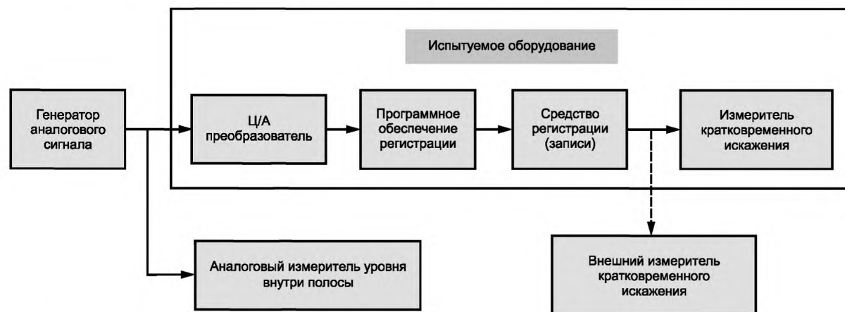
Рисунок 16 — Блок-схема для измерения кратковременных искажений
