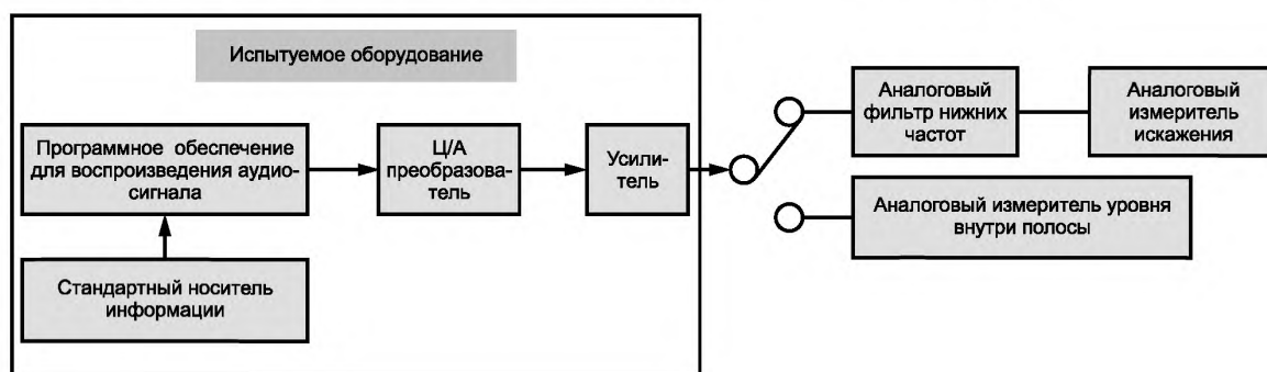
Рисунок 1 — Блок-схема для измерения максимальной амплитуды выходного сигнала
