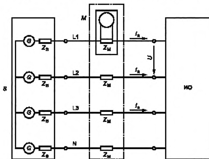
Рисунок А.1 — Схема измерений для однофазного оборудования
