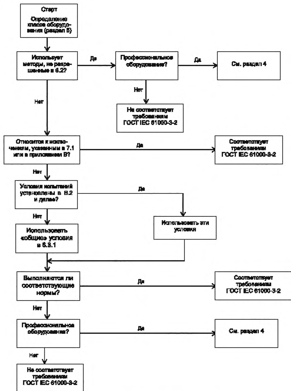
Рисунок 1 – Алгоритм для определения соответствия
