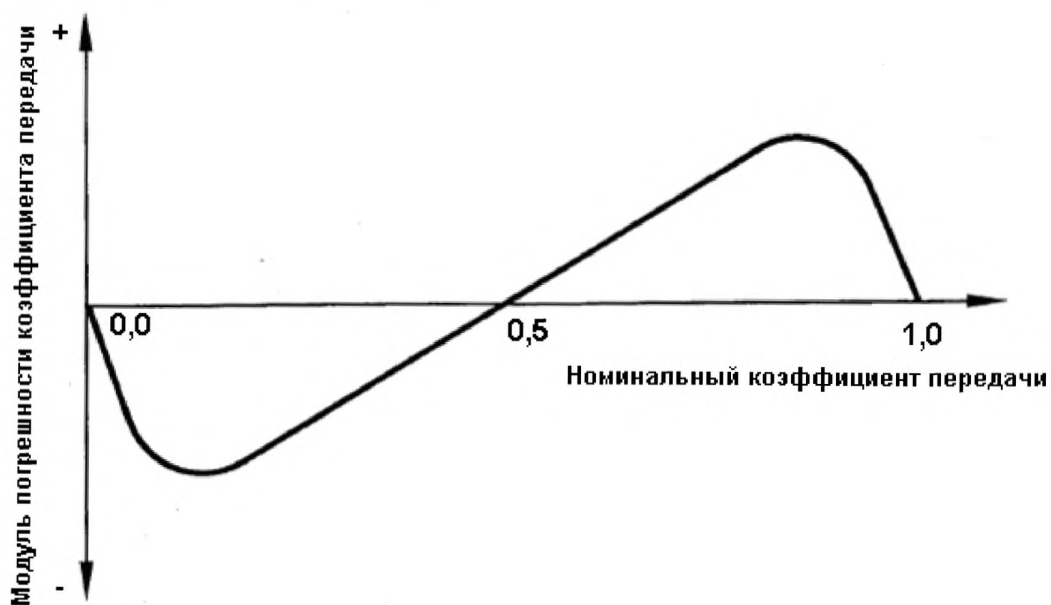
Рисунок 1 – Типовые погрешности коэффициента передачи
