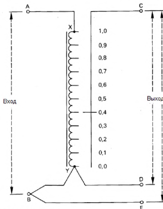
Рисунок 2 – Соединения входа и выхода индуктивного делителя напряжения
